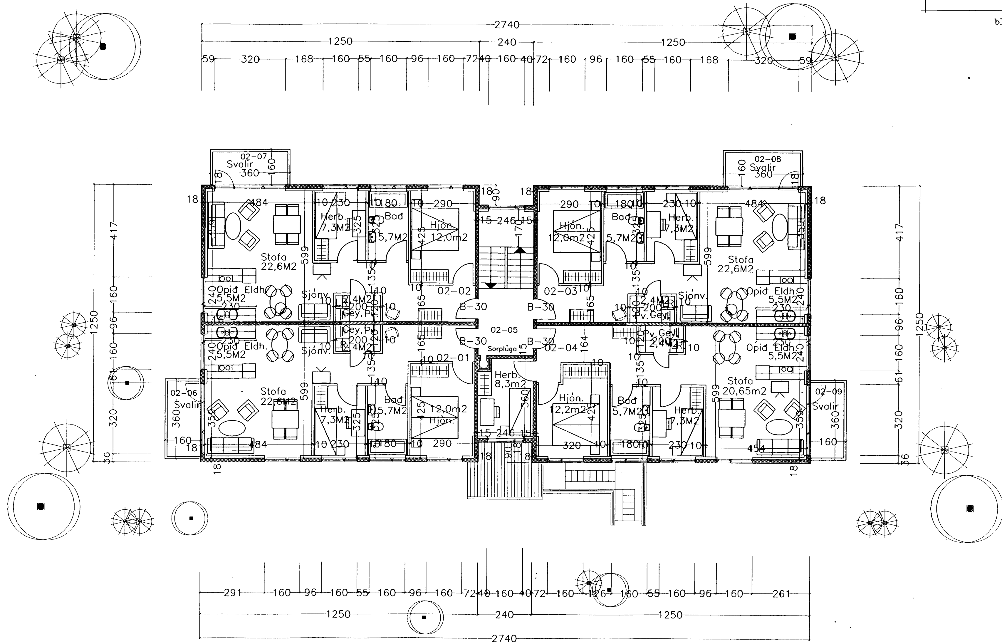
Grunnmynd 2 hæðar.
