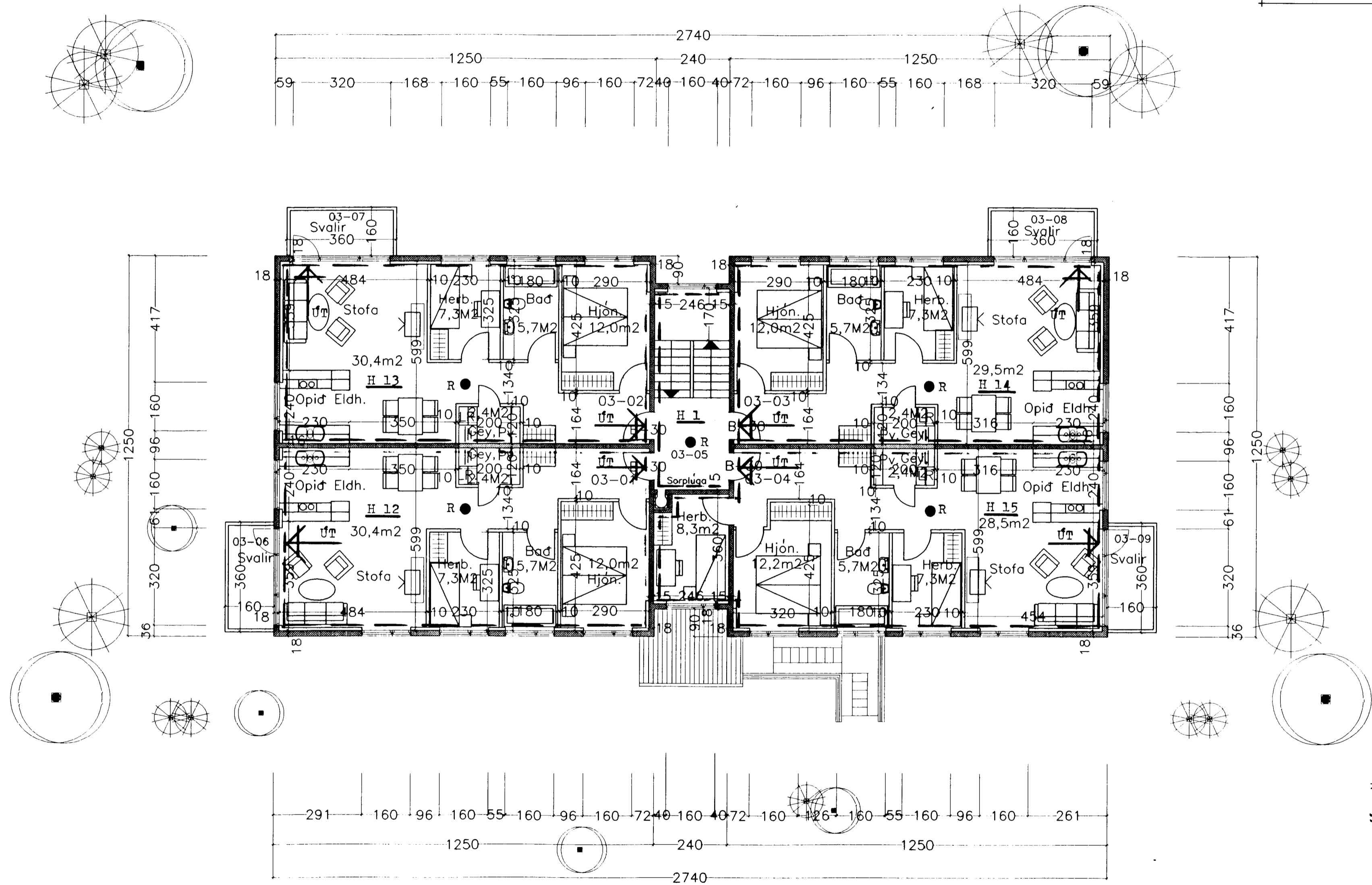
Grunnmynd 3 hæðar.
