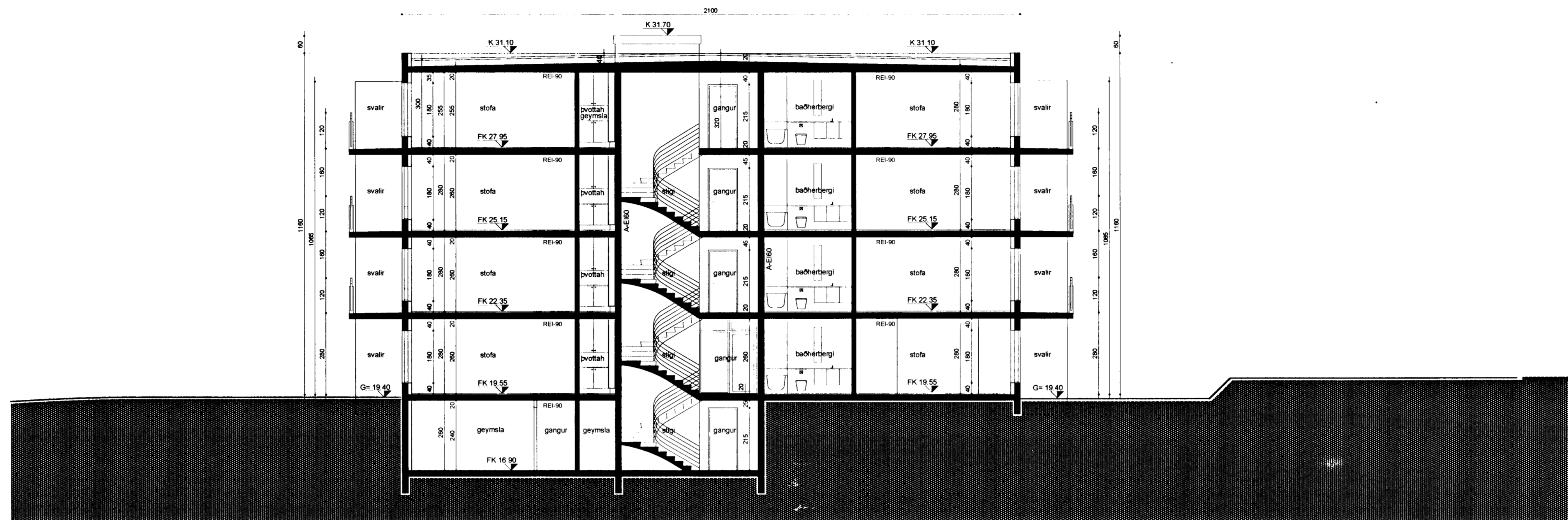
SNEIÐING AA
