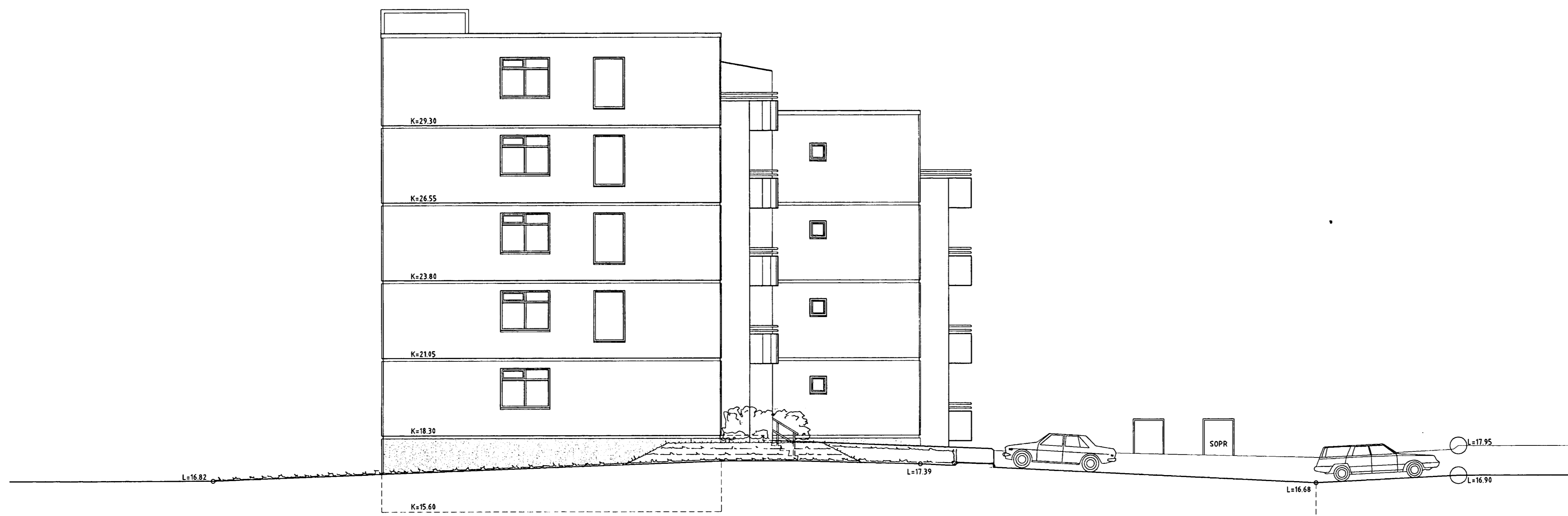
VESTURHLIÐ Mkv 1:100
