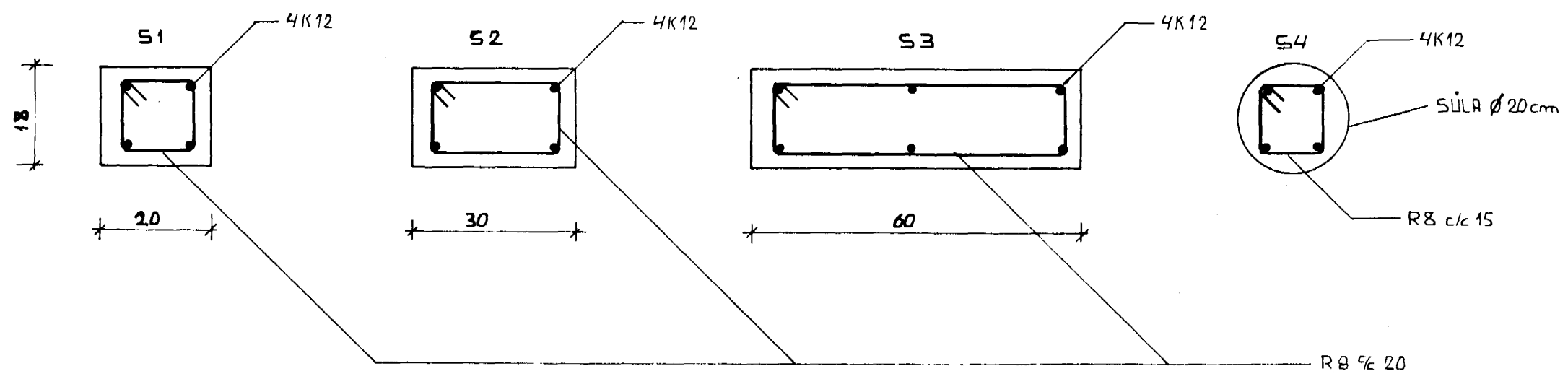
SÚLUR MKV 1:10
