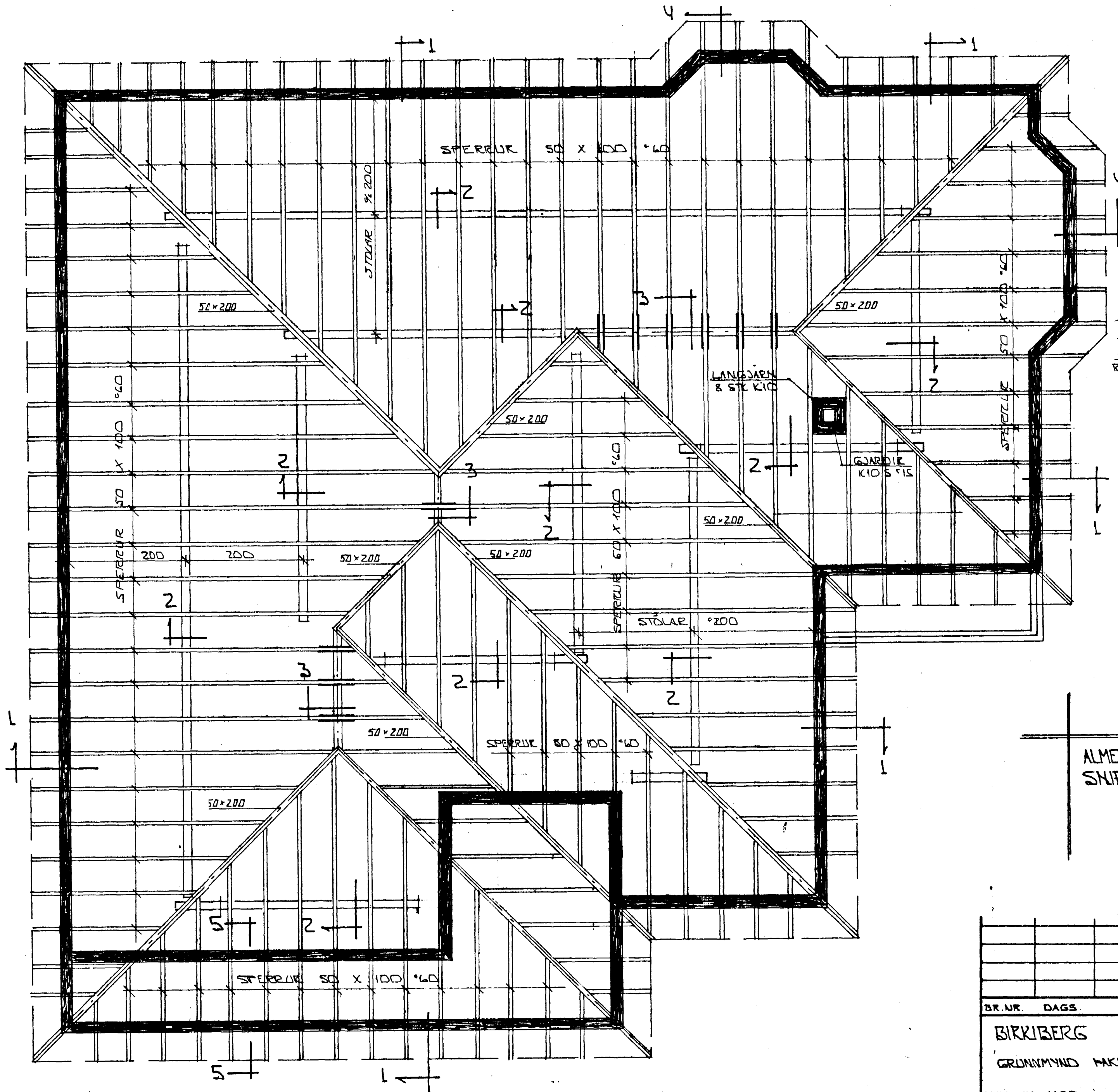
GRUNNMYND · 1:50
