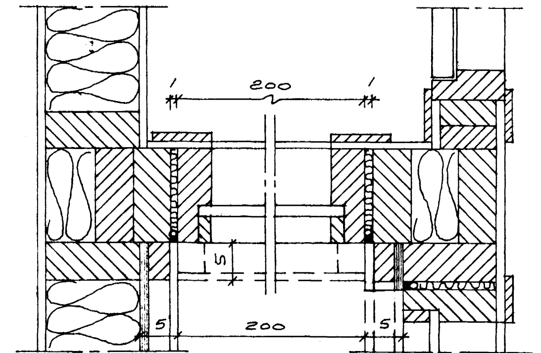
LÆRÉTT SNID Í ÚTIHURD KVOTTAKLISS, M=1:15
