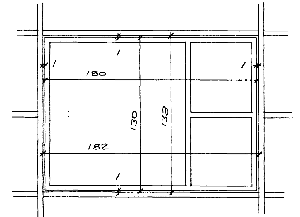
GLUGGI Í GRIND, M=1:20
