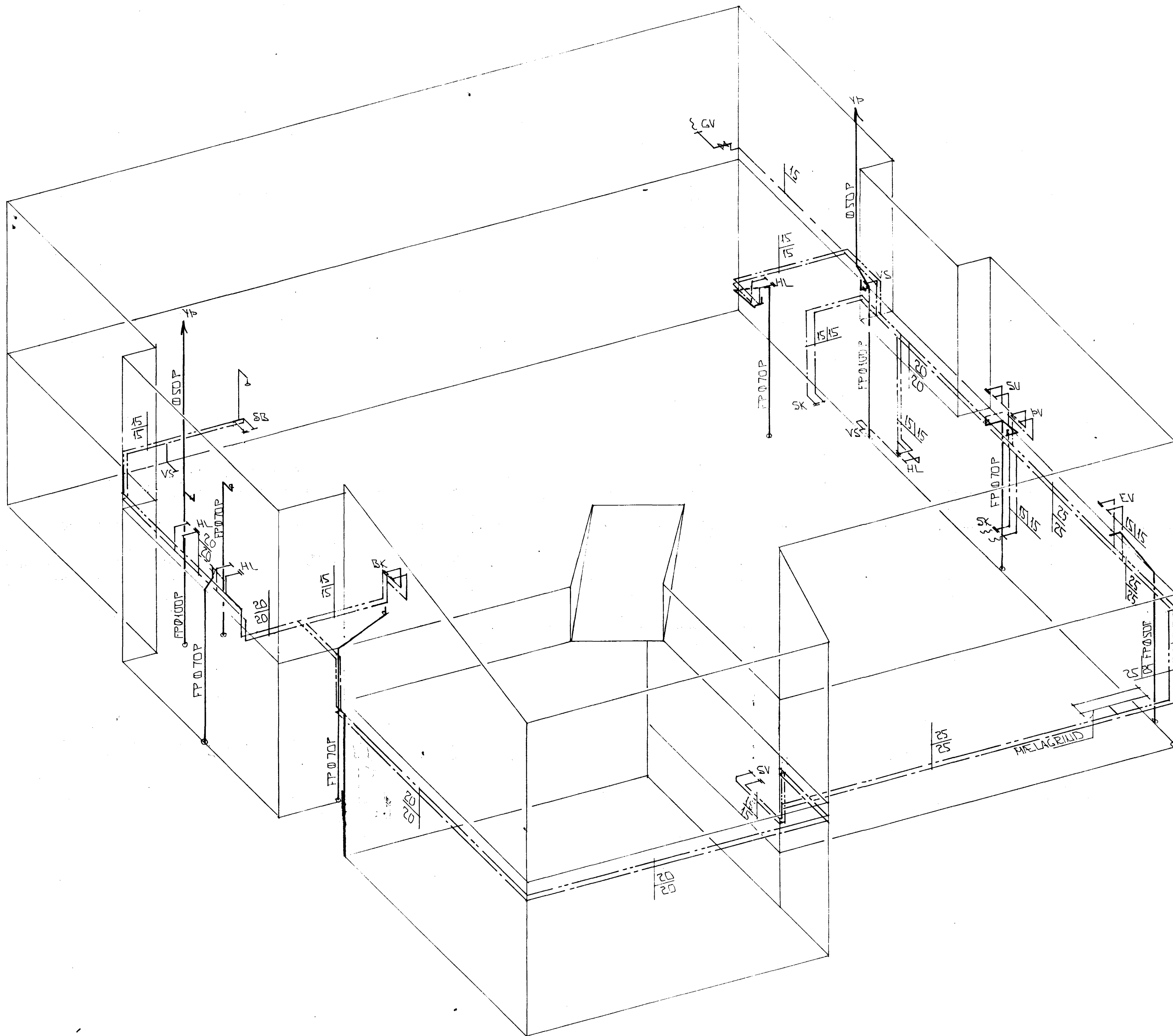
RÚMMYND - VATNSLAGNA 1:50
