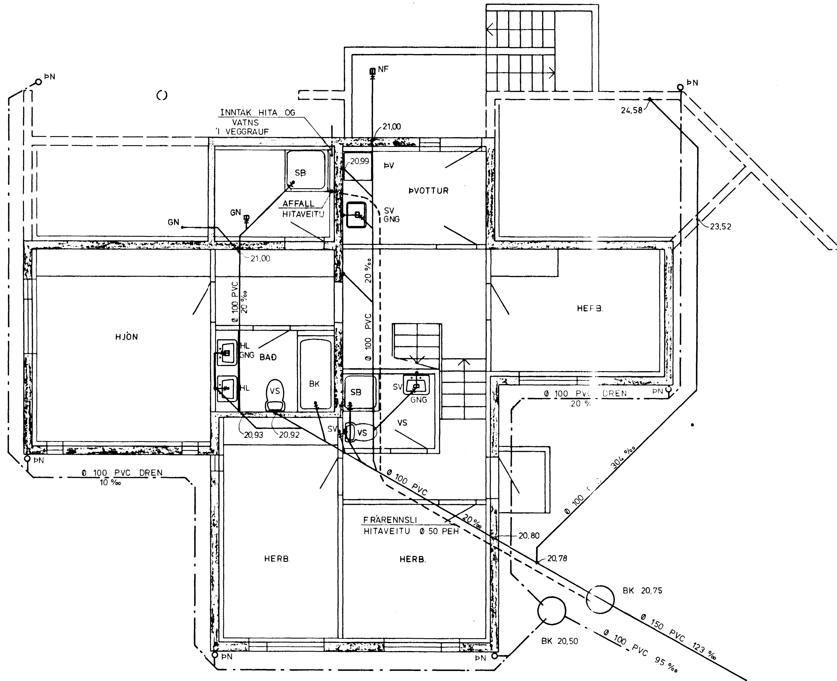
GRUNNMYND JARÐHÆÐAR 1:50
