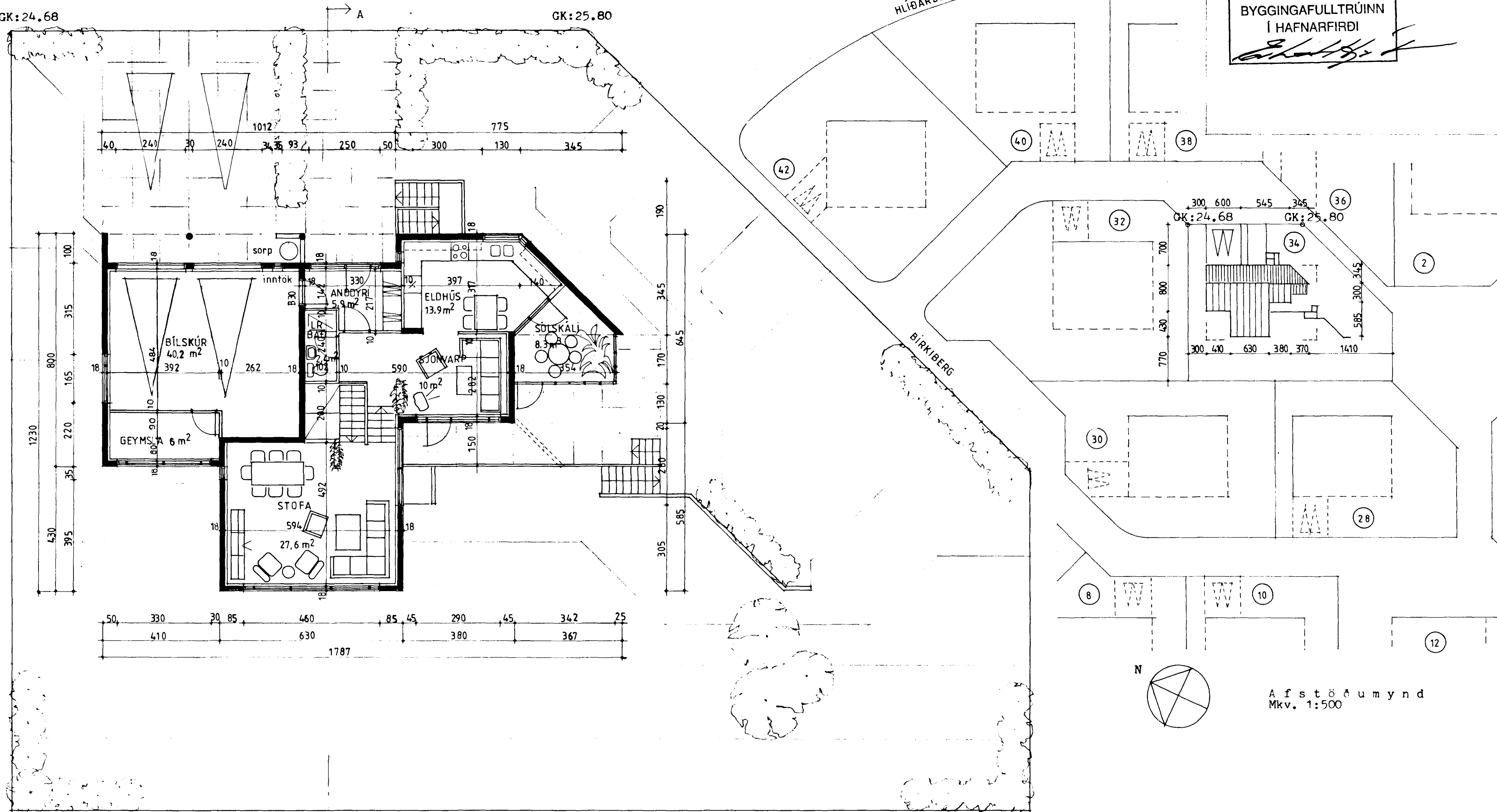
Grunnmynd aðal hæðar Mkv. 1:100
