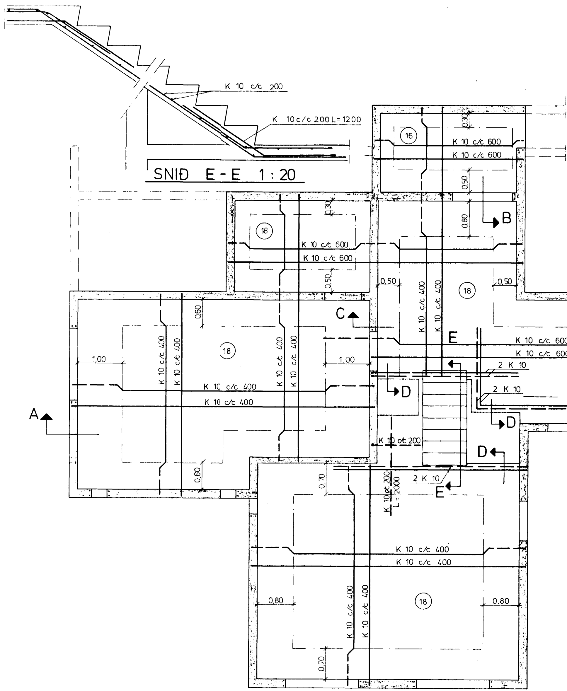
GRUNNMYND JARDHÆÐAR 1:50
