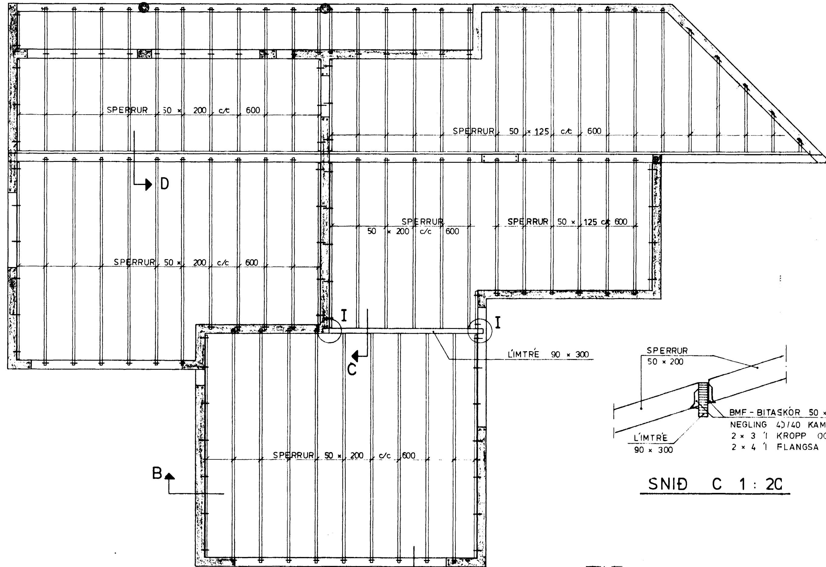
GRUNNMYND 1:50
