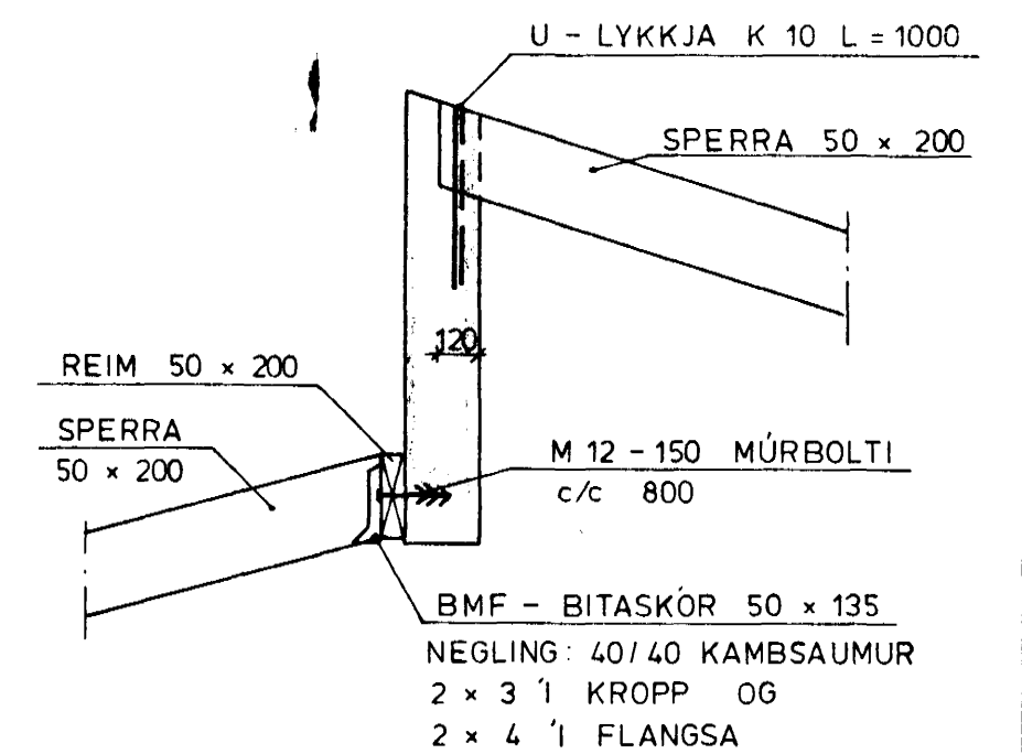
SNID D 1:20
