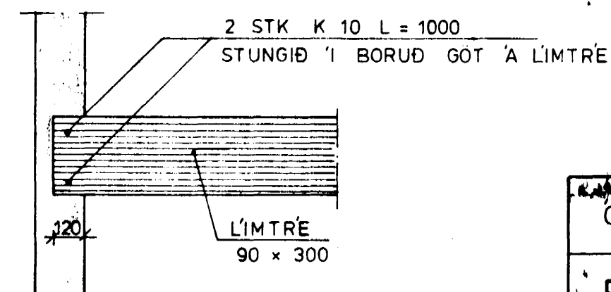
SÉRMYND I 1:20
