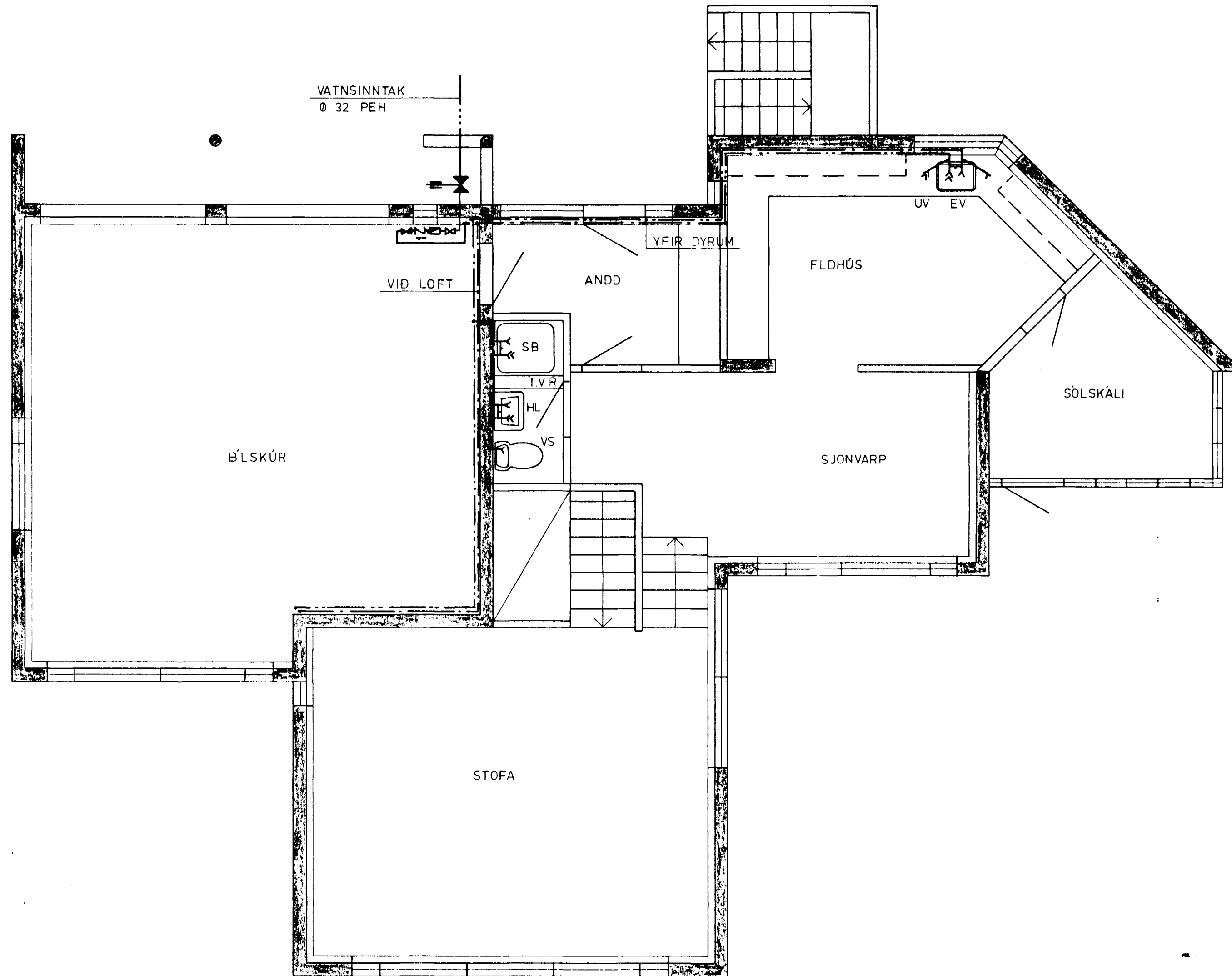
GRUNNMYND AÐALHÆÐAR 1 : 50
