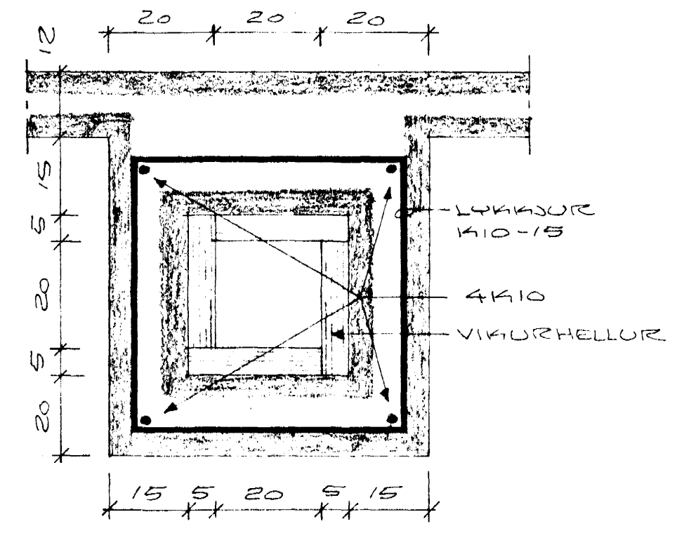
LÄRETT SNID Í REYKHÄF, M=1:10
