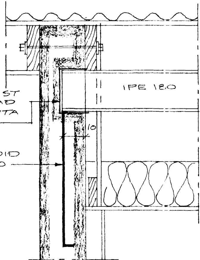
FESTING Á STÄLBITAENDAN Í VEGGI, M=1:10
