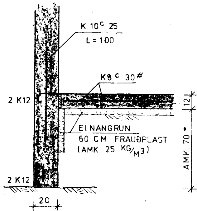
SNID 1-1 1:20
