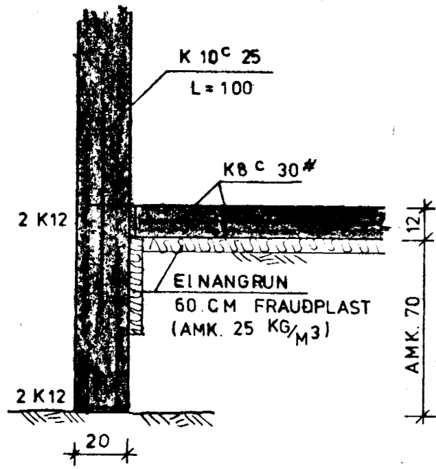
SNID 1-1 1:20
