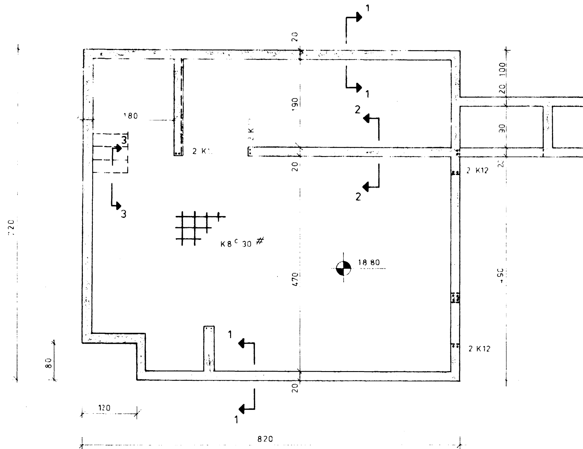
GRUNNMYND 1:50
