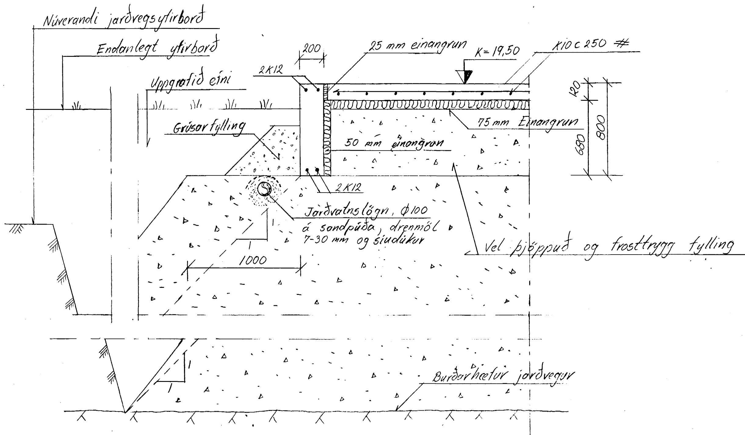
F Sníð: Málteikning, Jarðvinna og Járn bending 1-01 Mkv. 1:20
