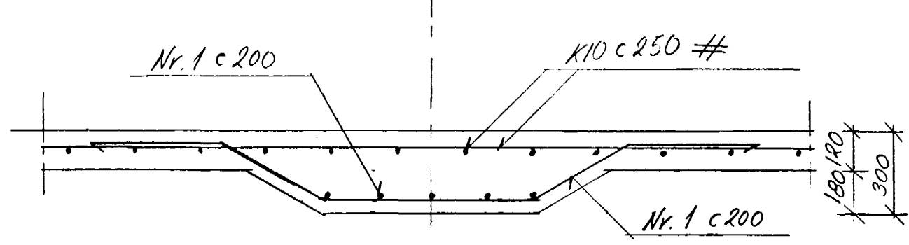
B Sníð: Járn bending 1-02 Mkv. 1:20
