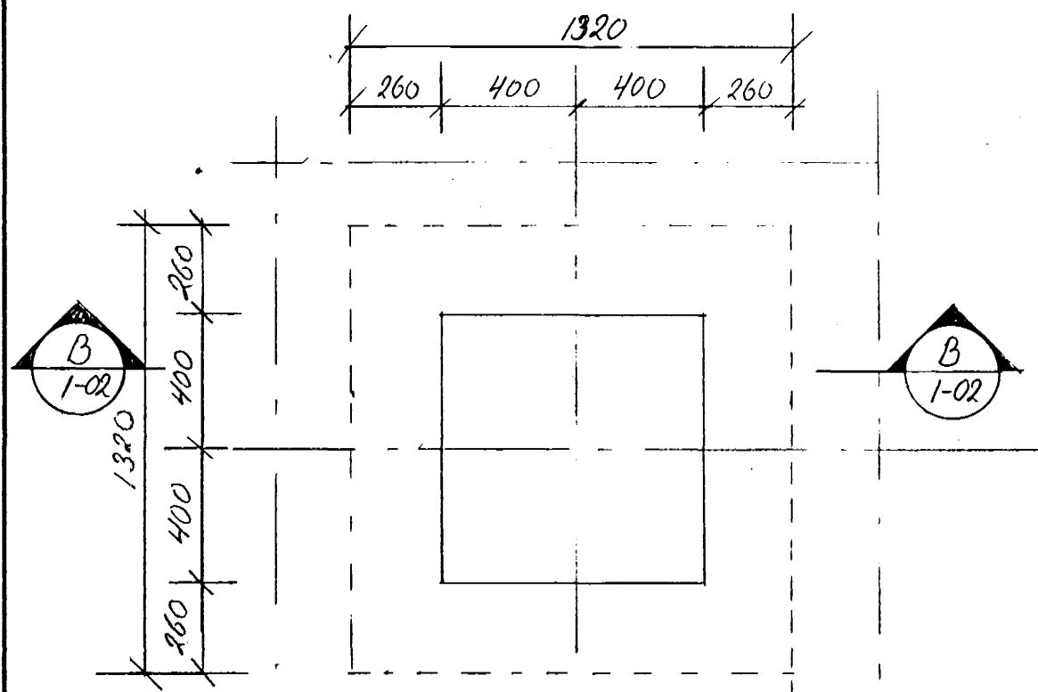
F Sníð: Málteikning, Jarðvinna og Járn bending 1-01 Mkv. 1:20
