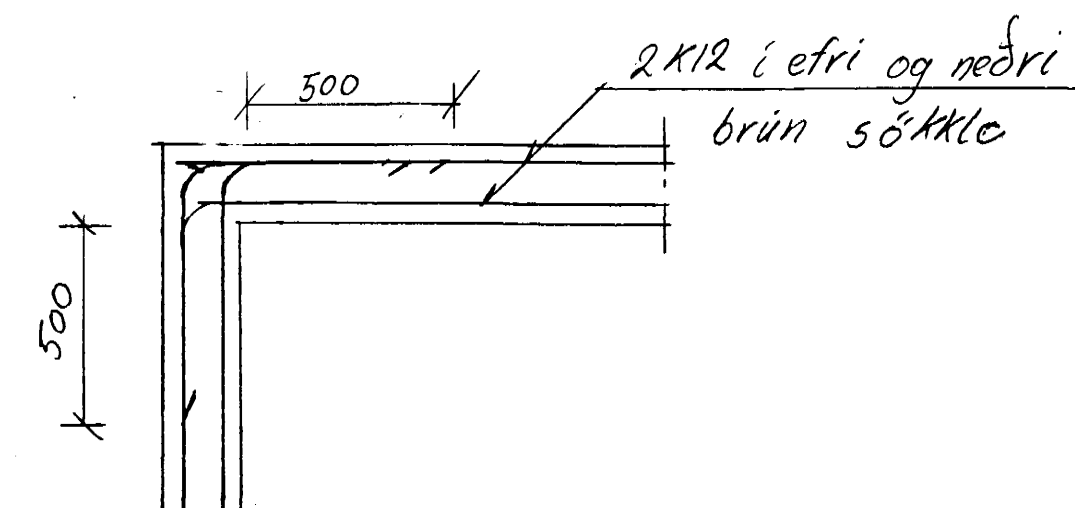
I Sérmynd I: Járn bending í hornum 1-01 Mkv. 1:20
