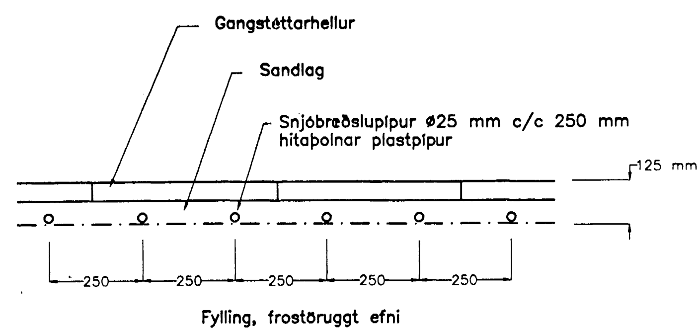
SNID Í SNJÓBRÆDSLUM. Mkv. 1:10
