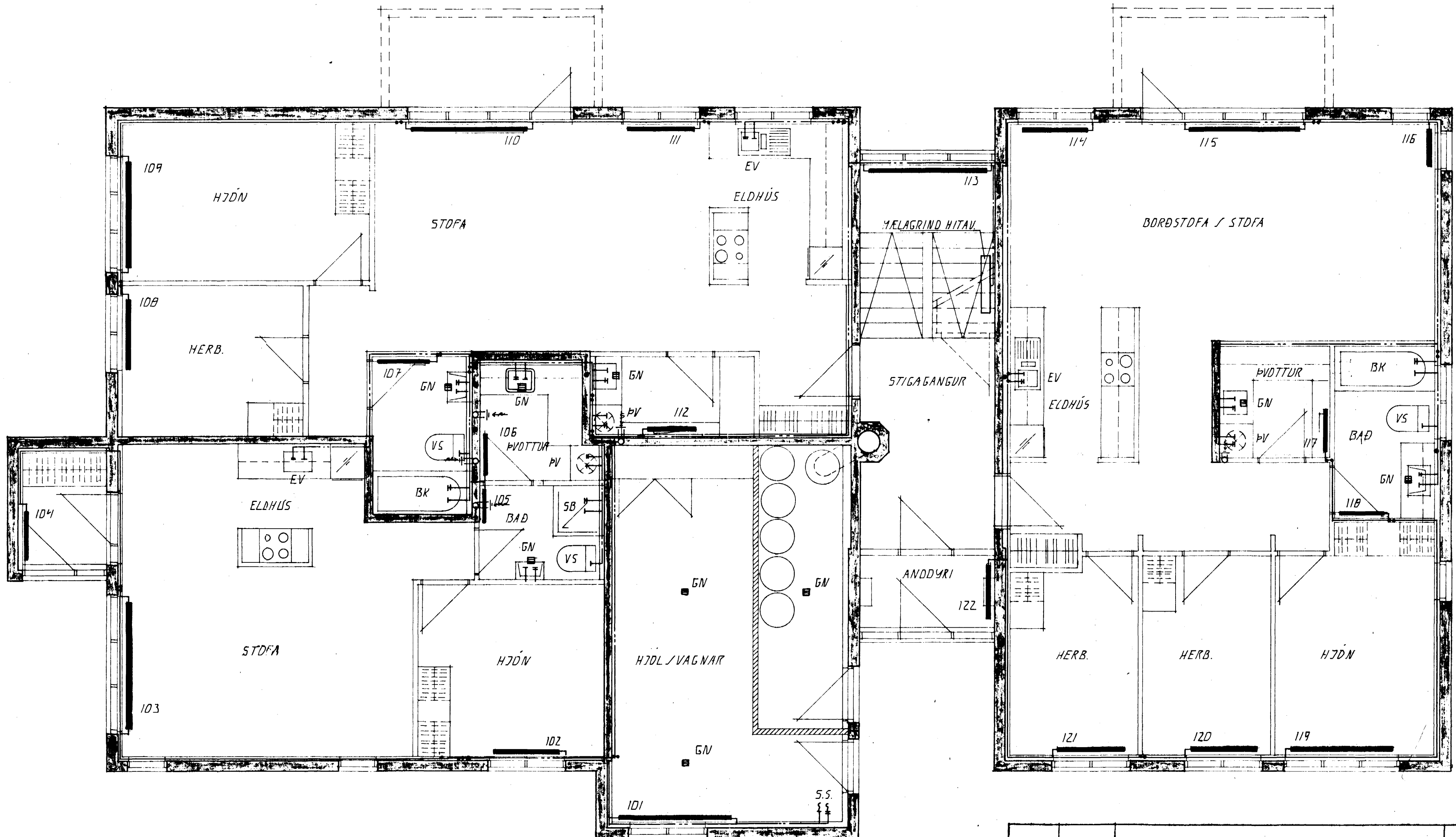
1. HÆÐ GRUNNMYND, 1:50
