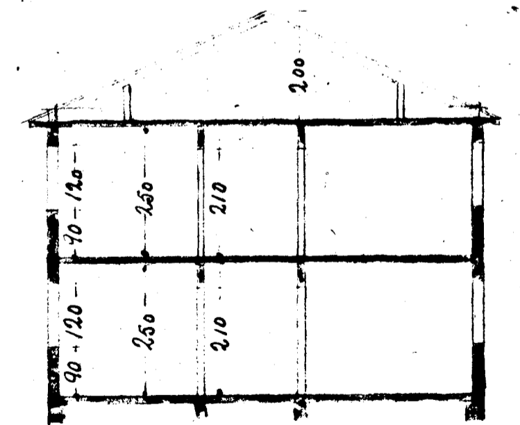
Þverskurður
