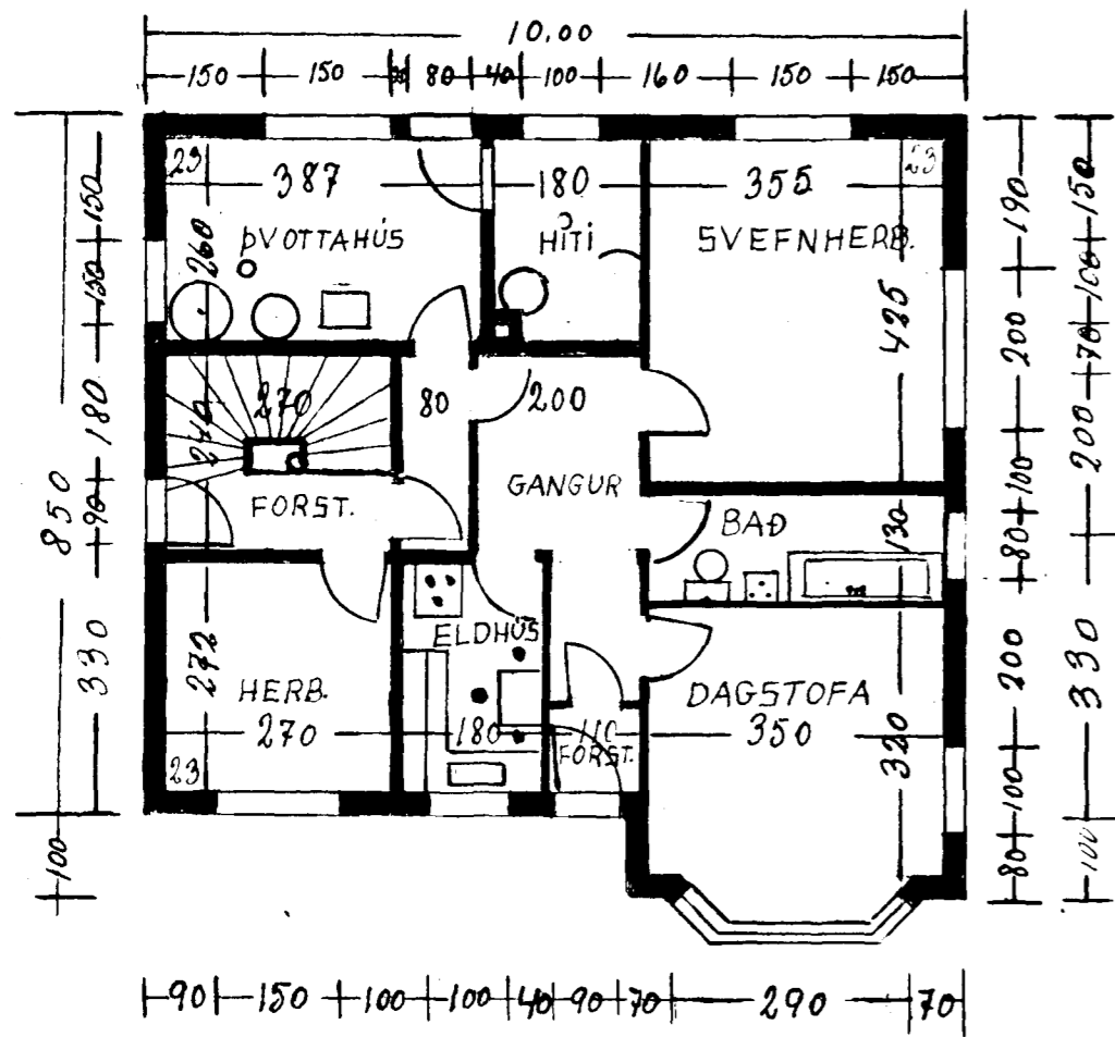
SUÐV.
