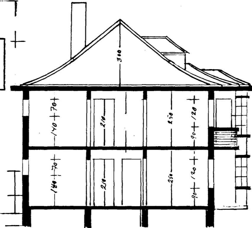
SKURÐUR A:A
