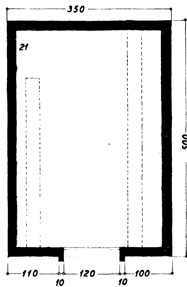
Grunnmynd
