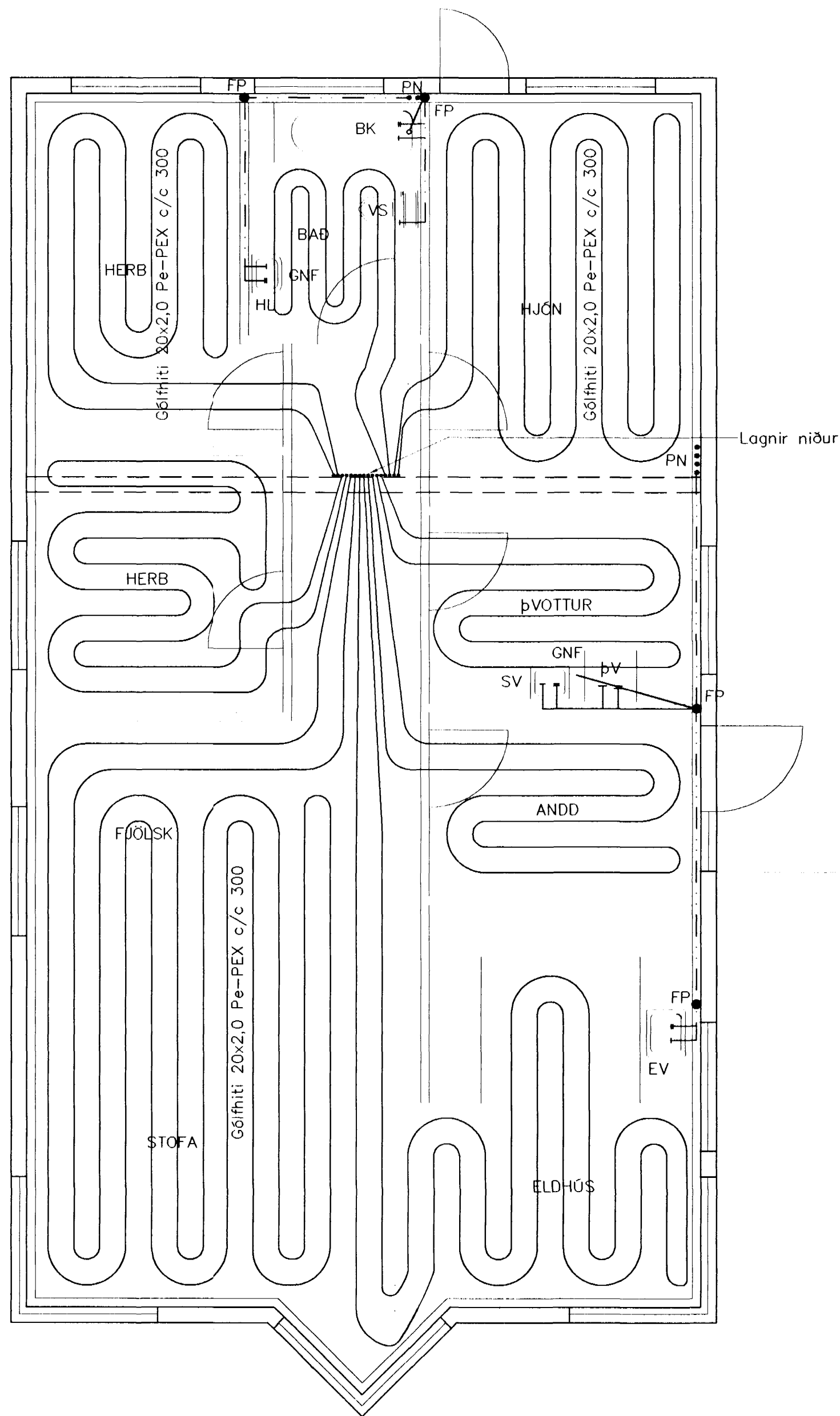
Grunnmynd 2. hæð, 1:50
