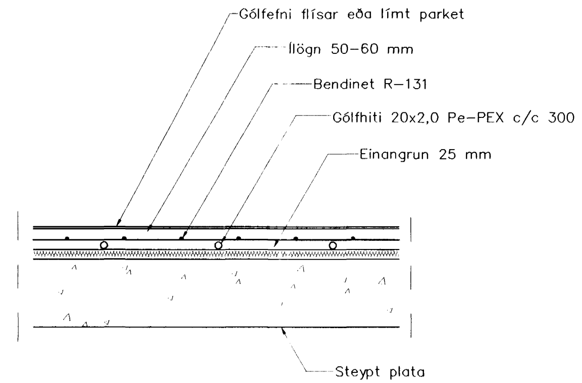
Gólfhiti snið, 1:10
