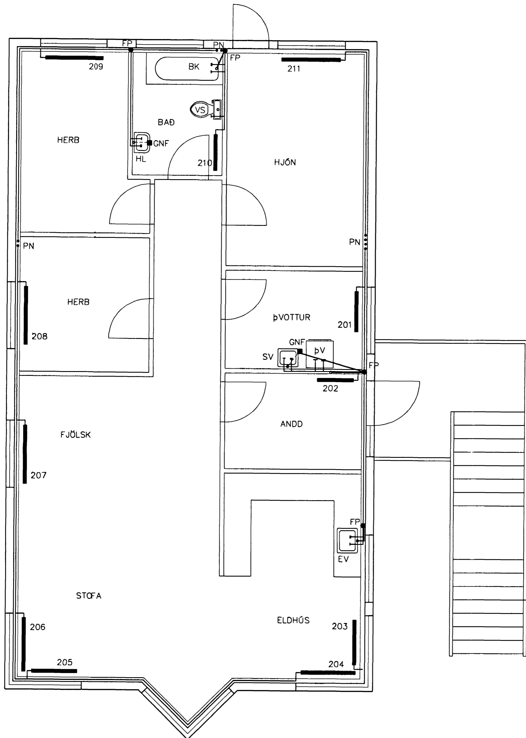
GRUNNMYND 2 HÆÐAR 1:50
