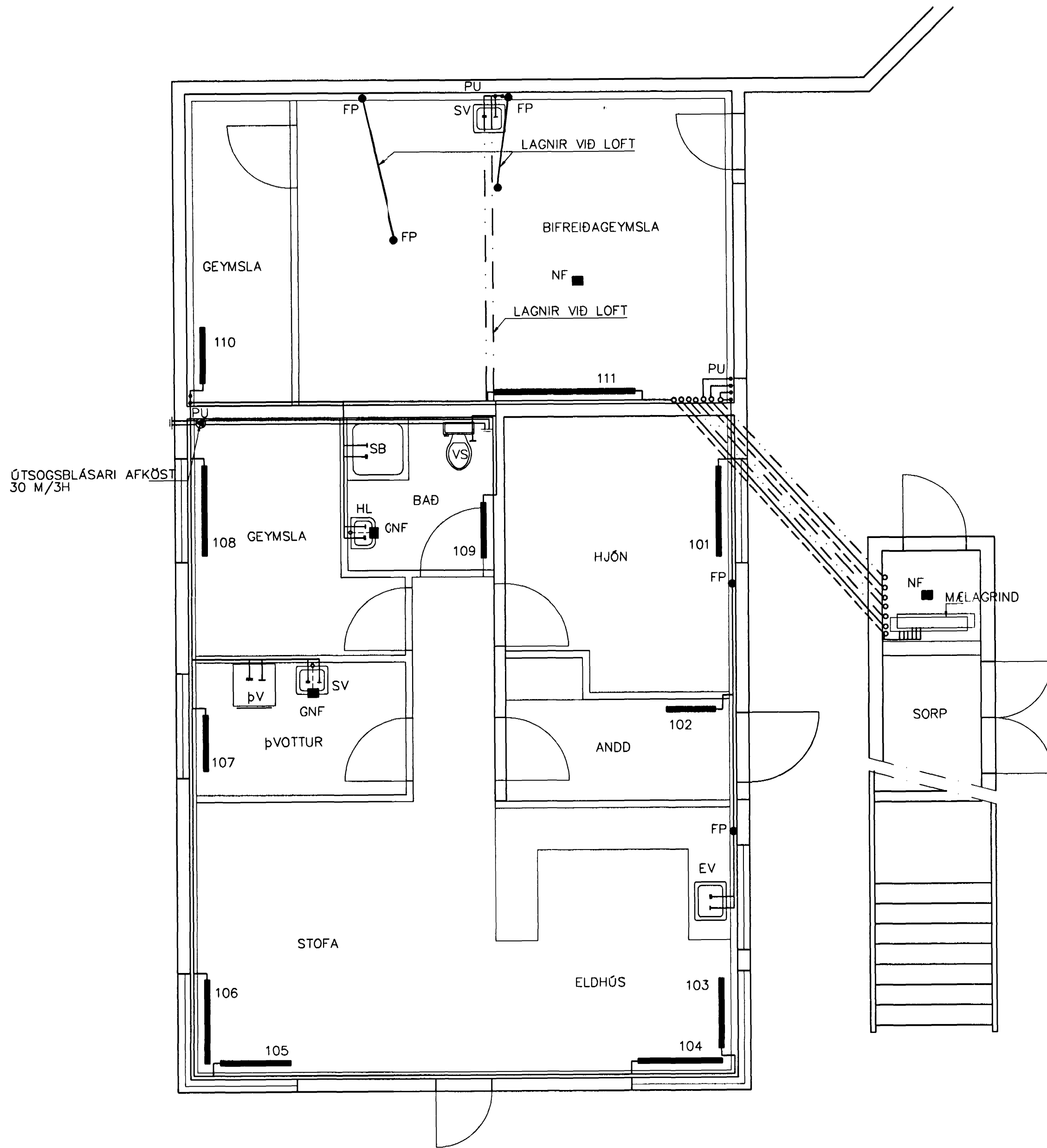
GRUNNMYND 1 HÆÐAR 1:50
