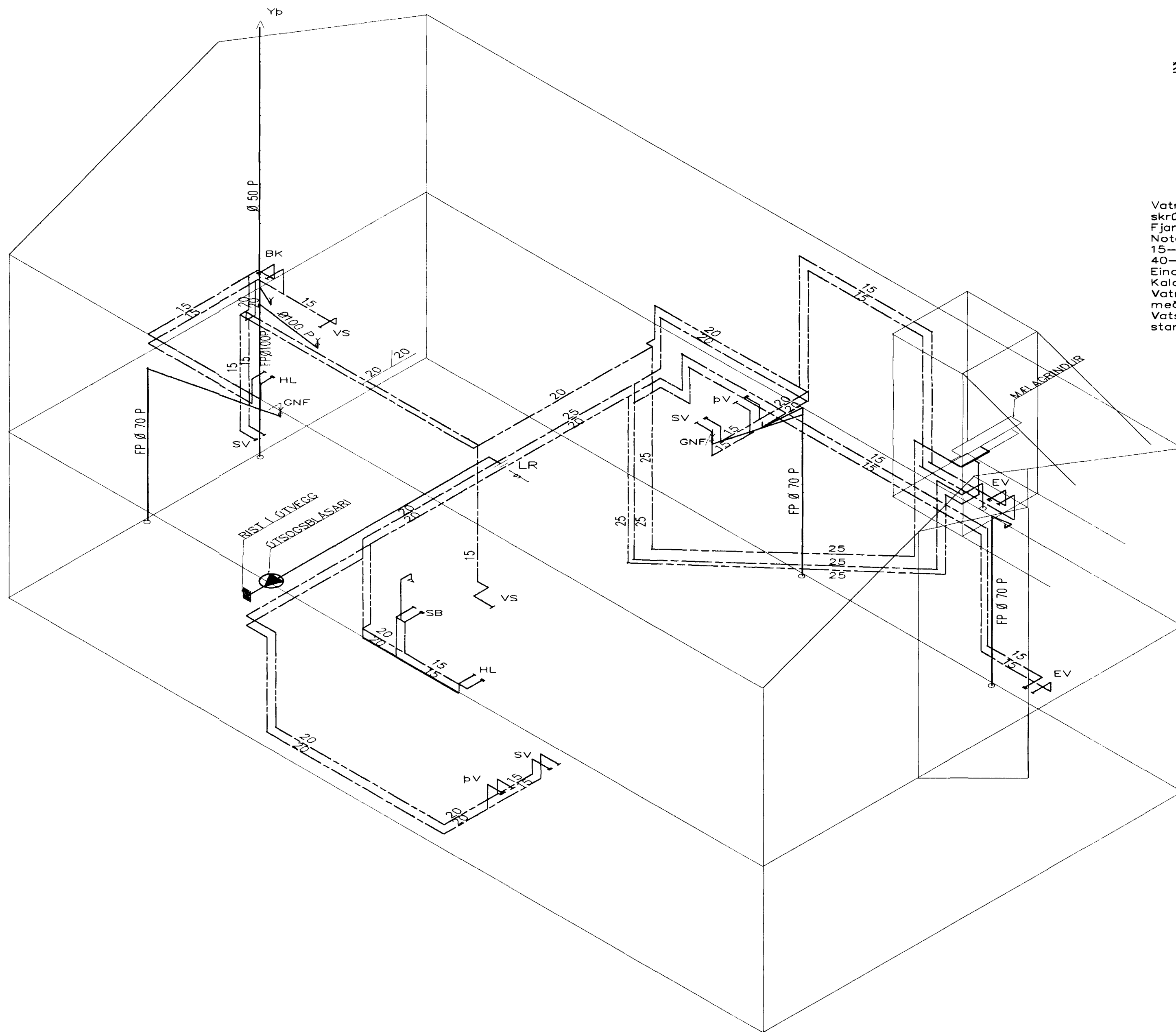
RÚMMYND VATNS OG FRÆRENNSLISLAGNA 1:50
