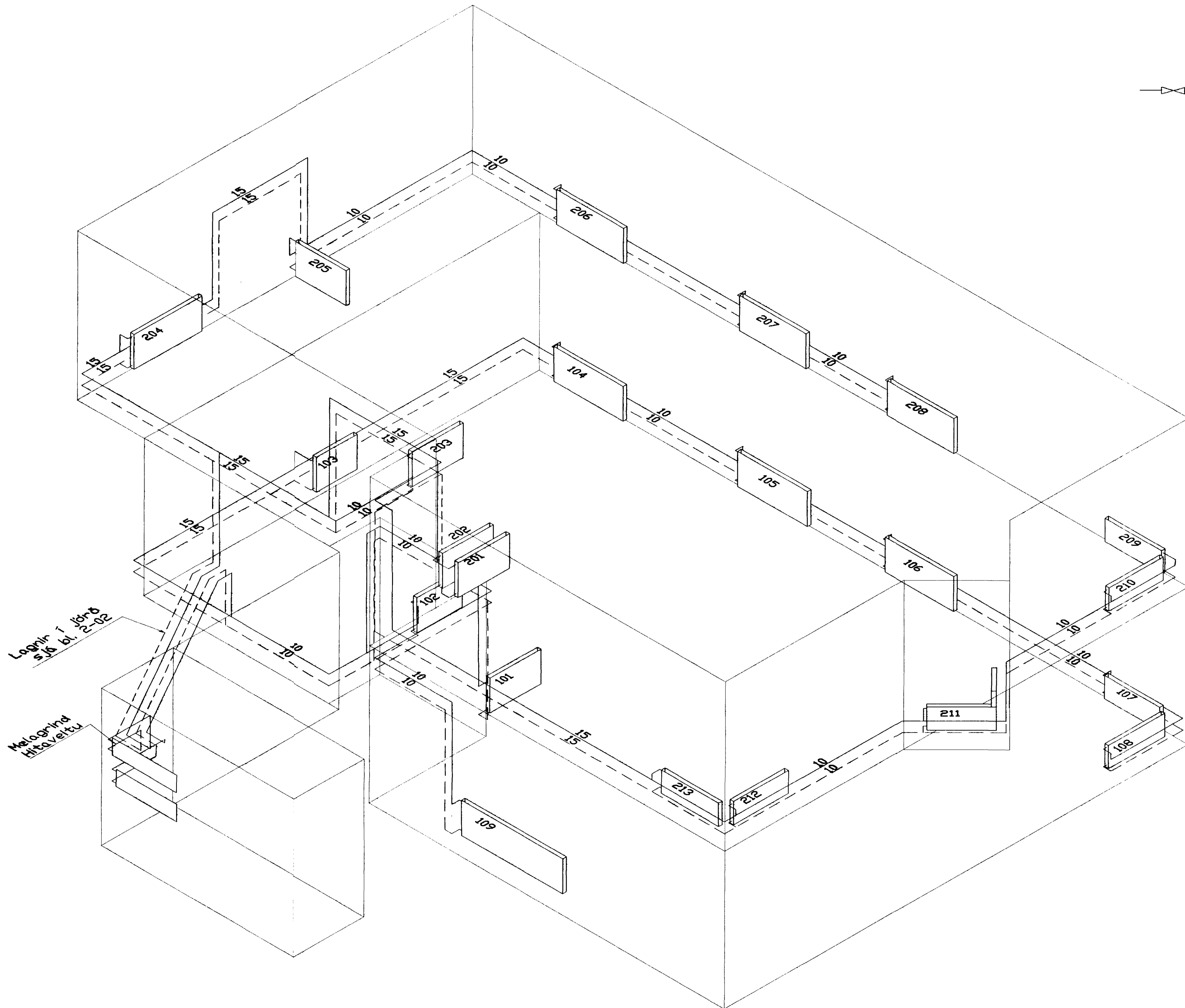
HITALAGNIR RÜMMYND, 1:50
