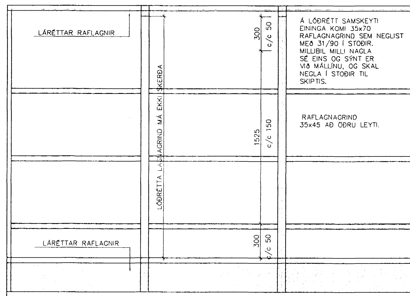
FRÁGANGUR RAFLAGNAGRINDAR 1:20
