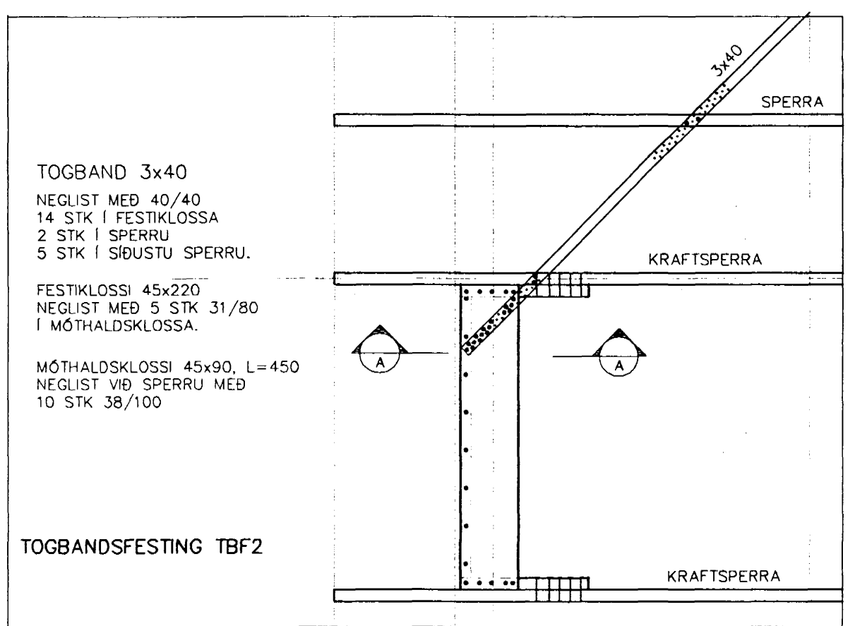
FESTING TOGBANDA Í ÞAKI 1:20
