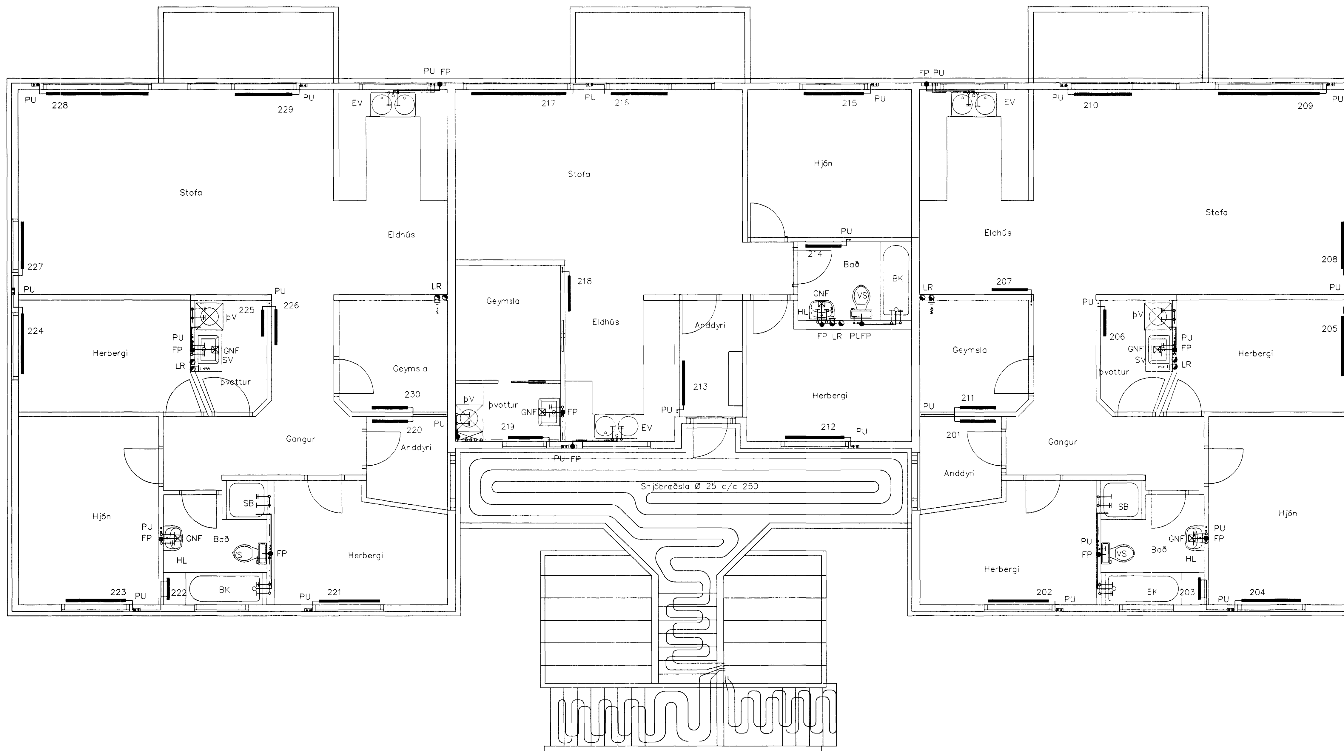
GRUNNMYND 2 HÆÐAR 1:50
