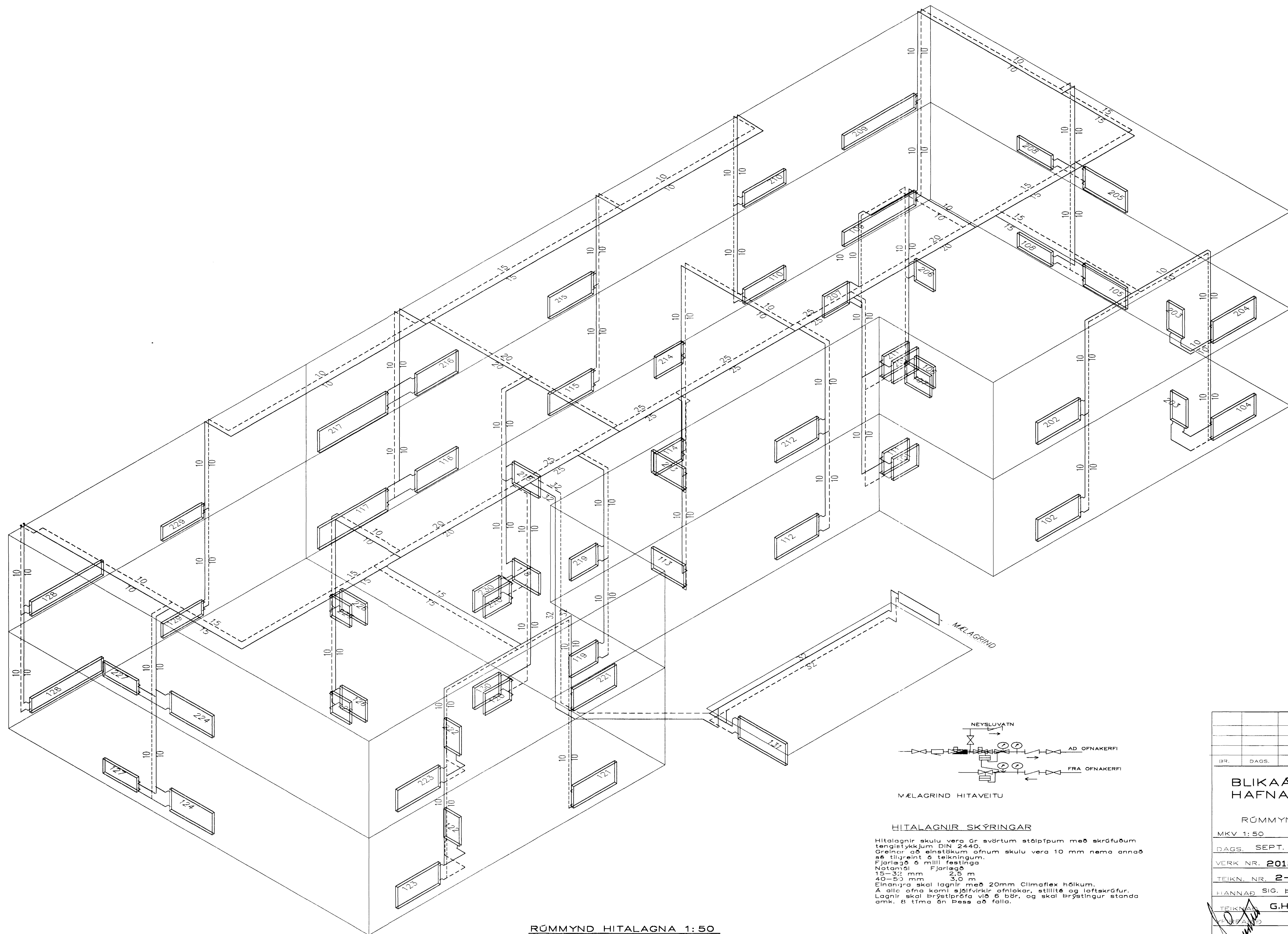
RÜMMYND HITALAGNA 1:50
