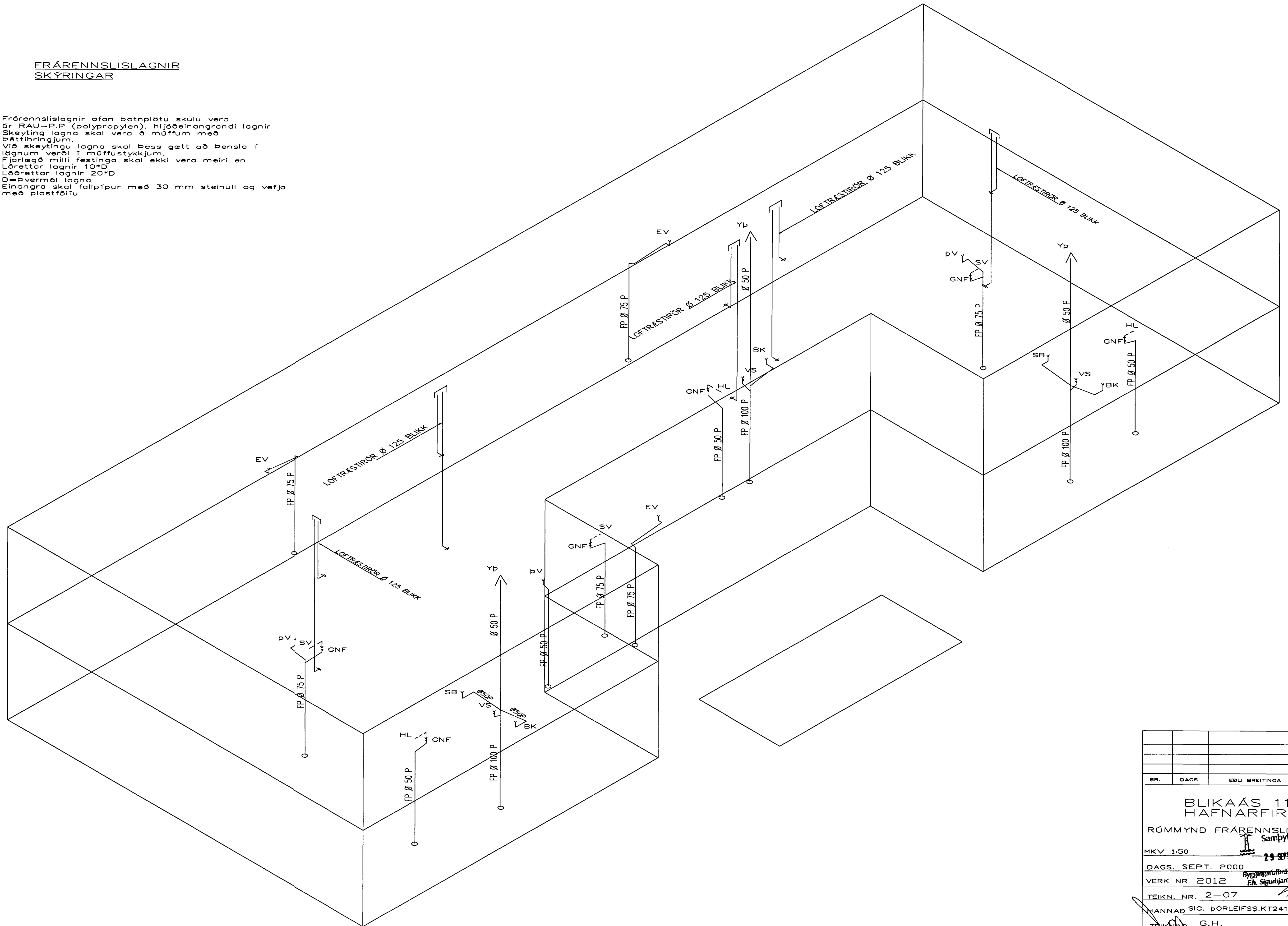
RÚMMYND FRÁRENNSLISLAGNA 1:50
