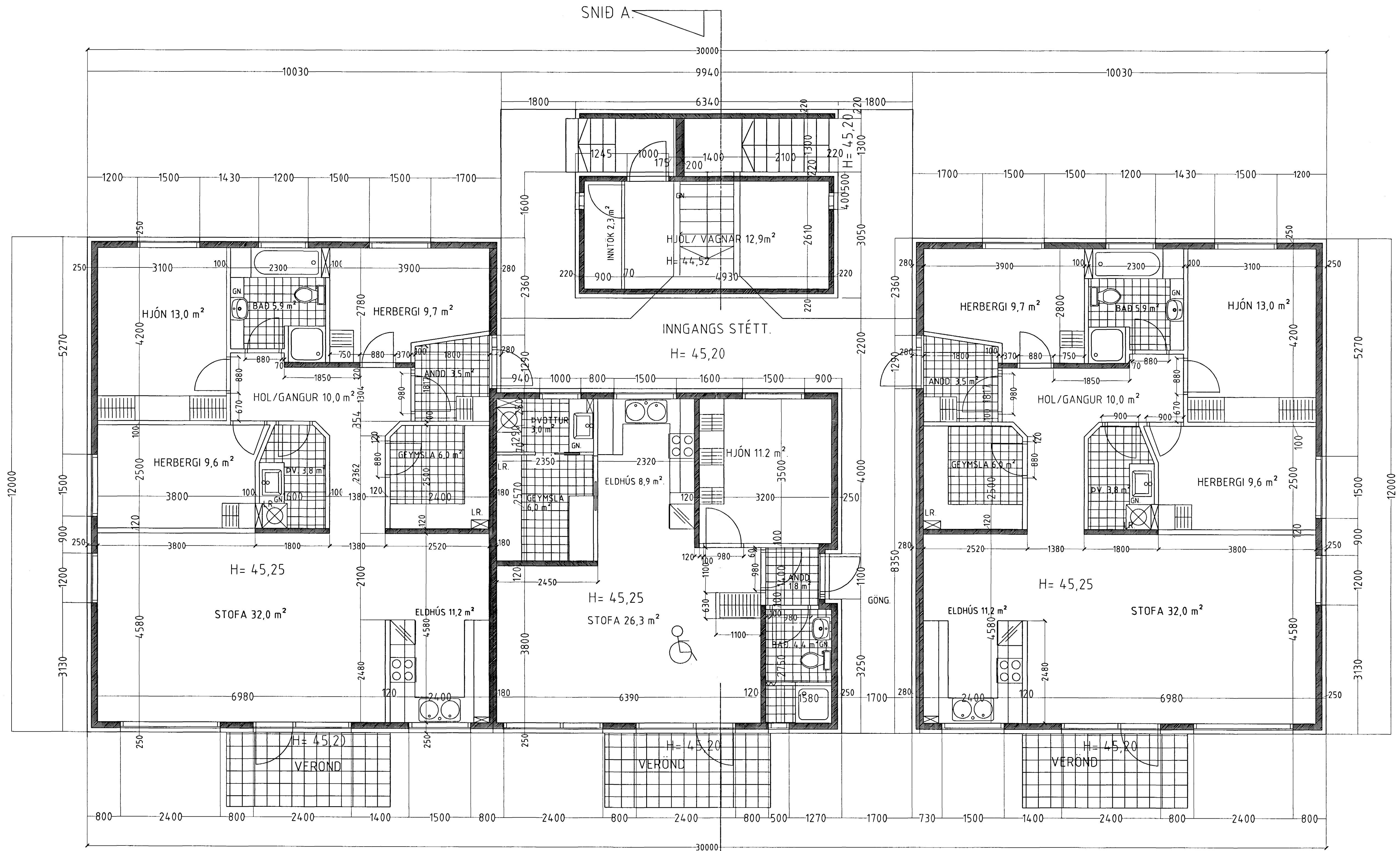
Grunnmynd 1. hæð. mkv. 1:50.
