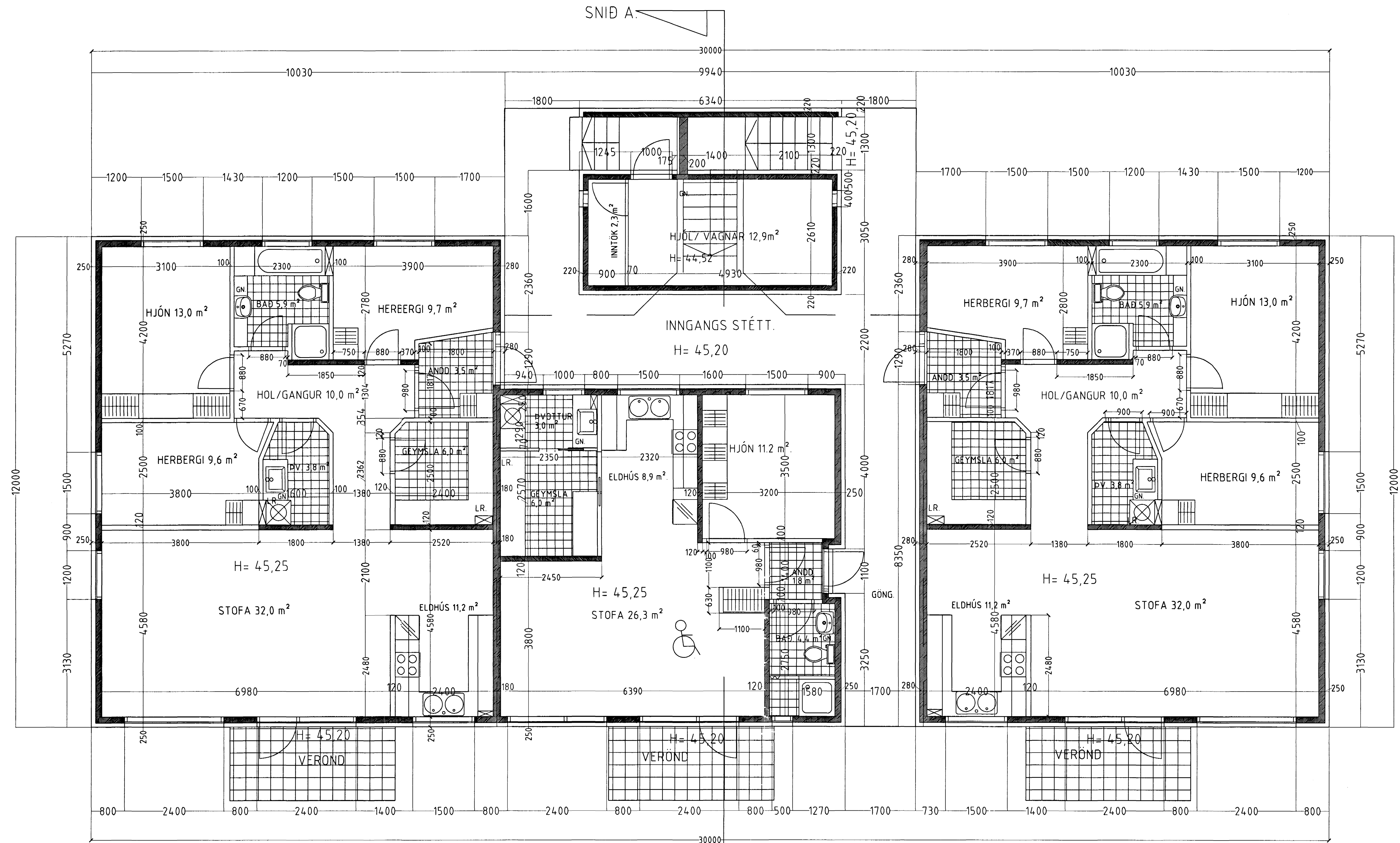
Grunnmynd 1. hæð. mkv. 1:50.
