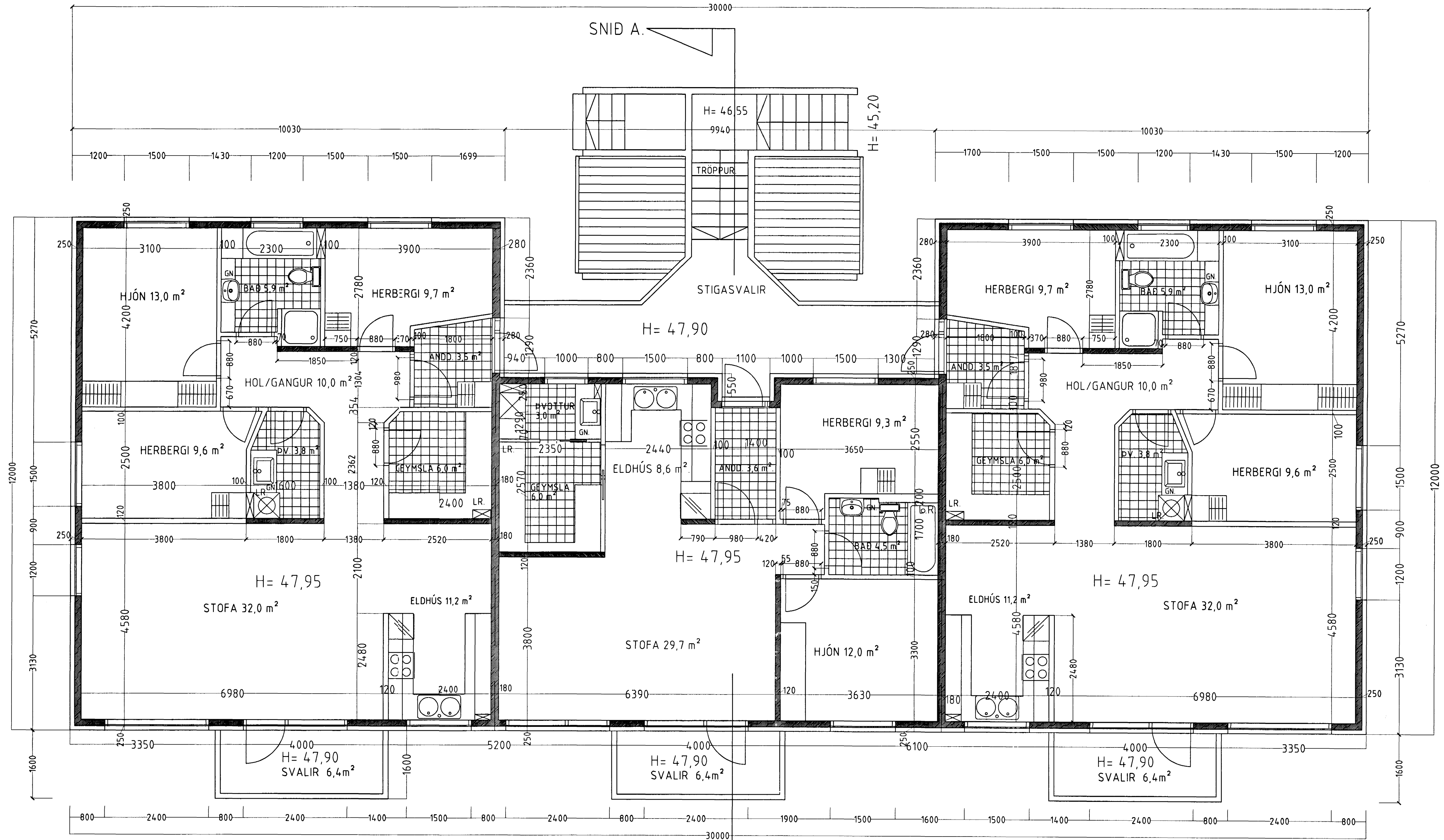
Grunnmynd 2. hæð. mkv. 1:50.
