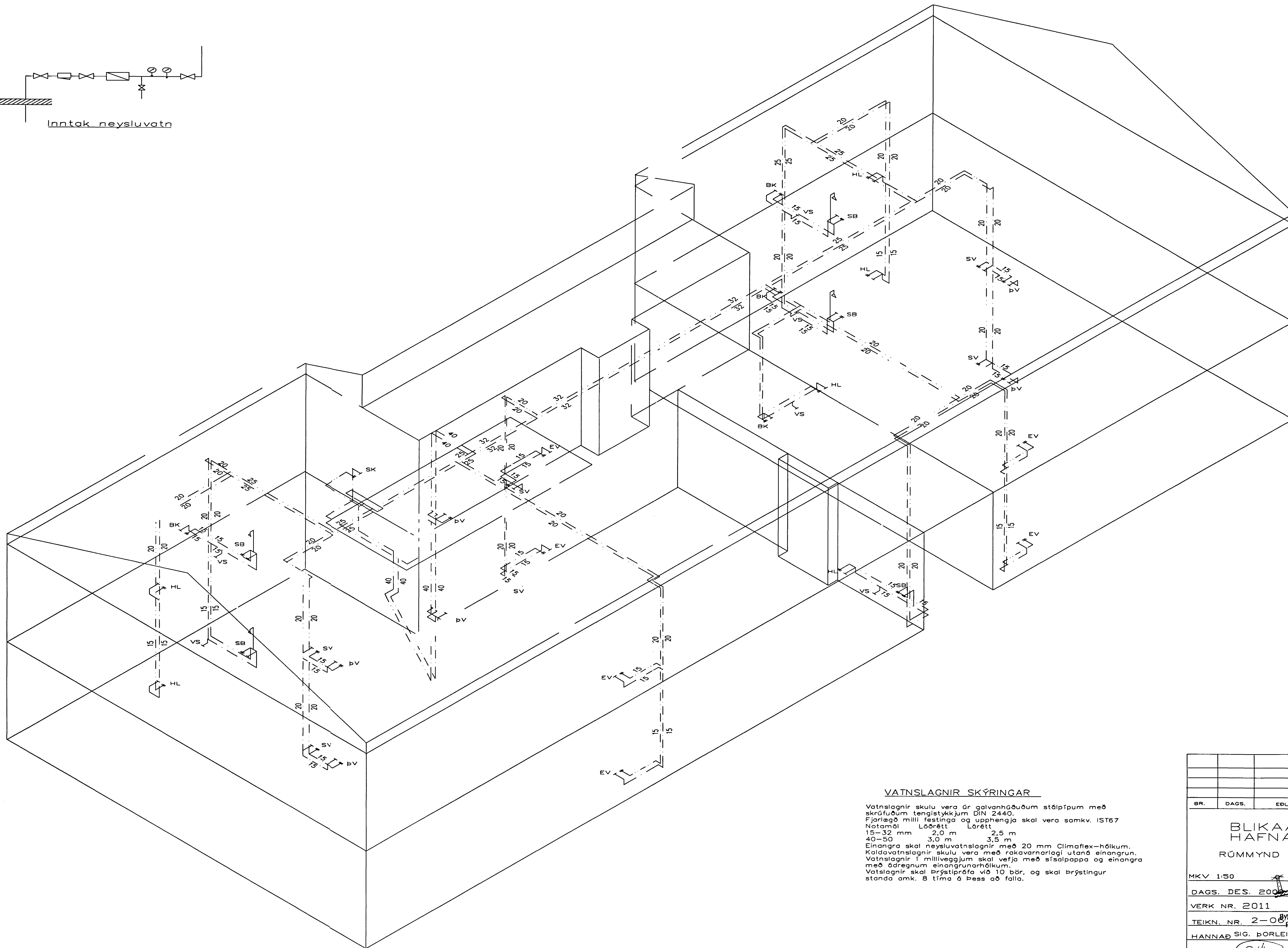
RÚMMYND VATNSLAGNA 1:50
