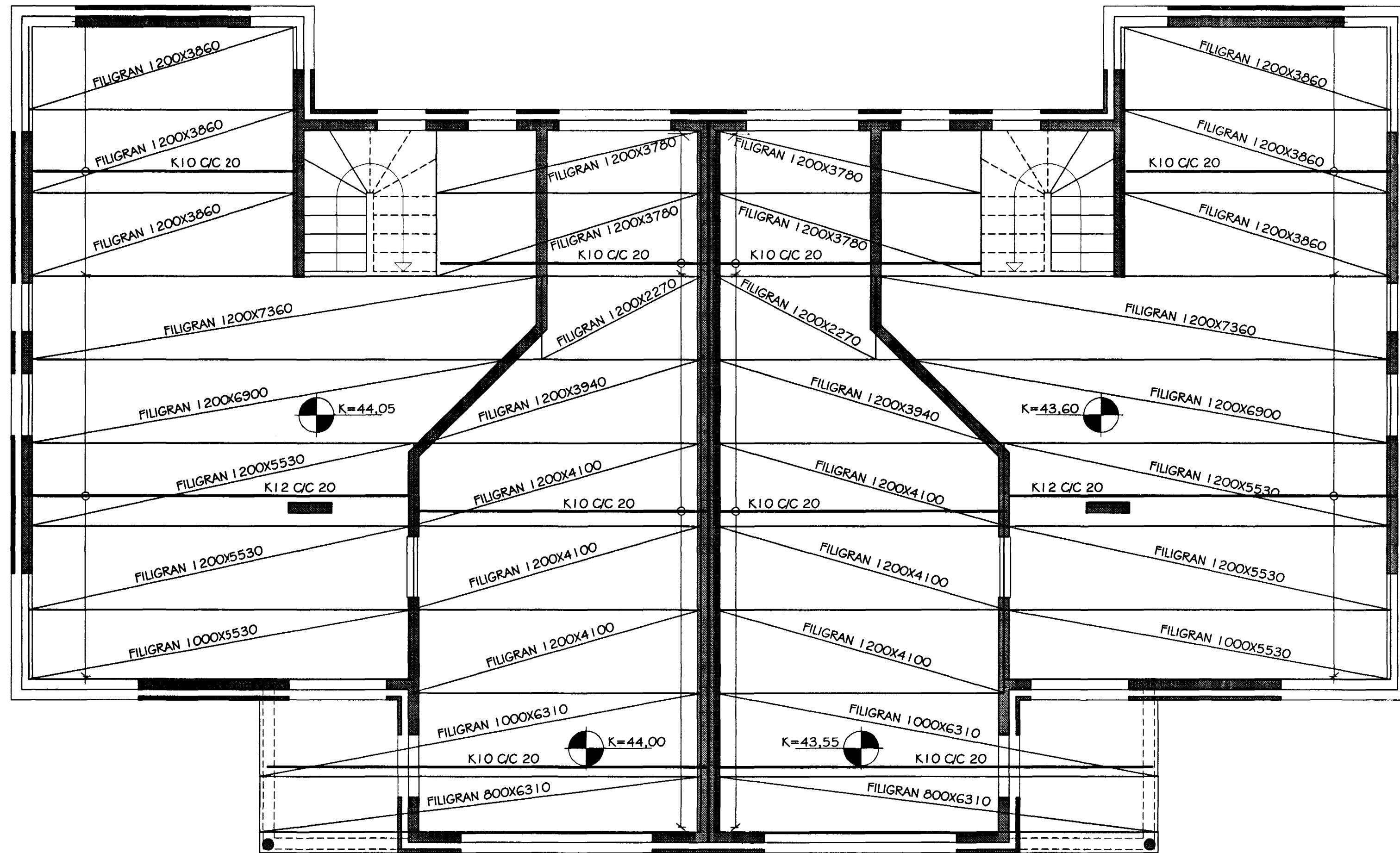
MILLIGÓLF - FORSTEYPTAR FILIGRANPLÖTUR GRUNNMYND MKV. 1:50
