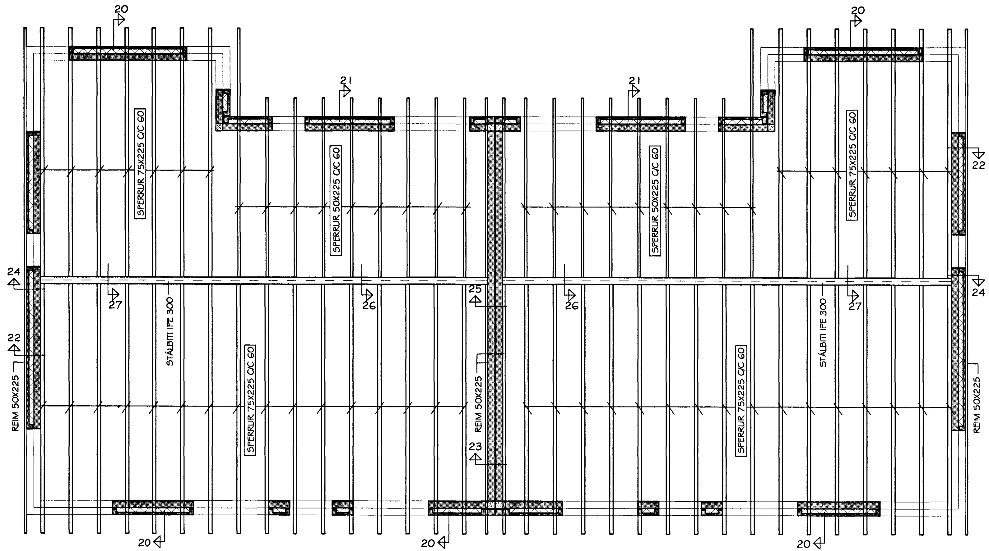
ÞAKVIÐIR GRUNNMYND MKV. 1:50
