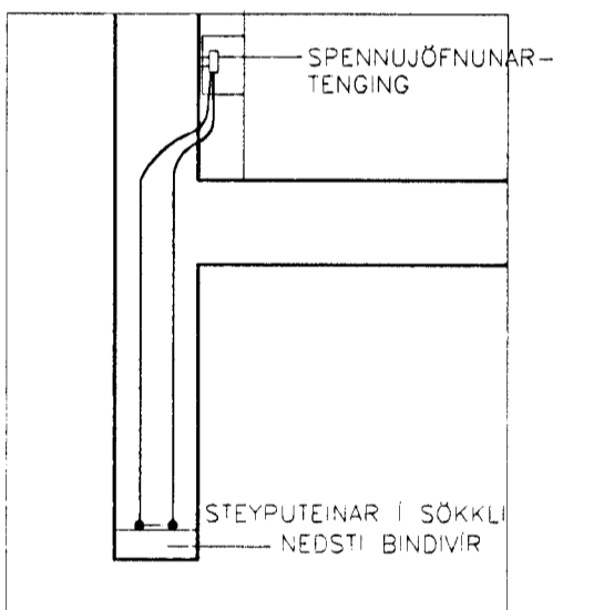
SNÍÐ AF TENGIÐI SÖKKULSSKAUTS
