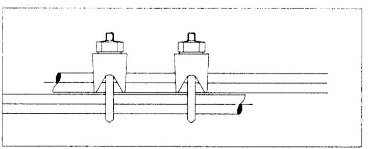
SNÍÐ AF TENGIÐI SÖKKULSSKAUTS
