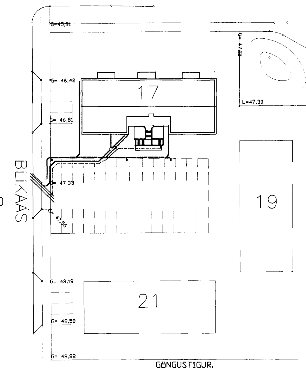
Afstöðumynd 1:500
