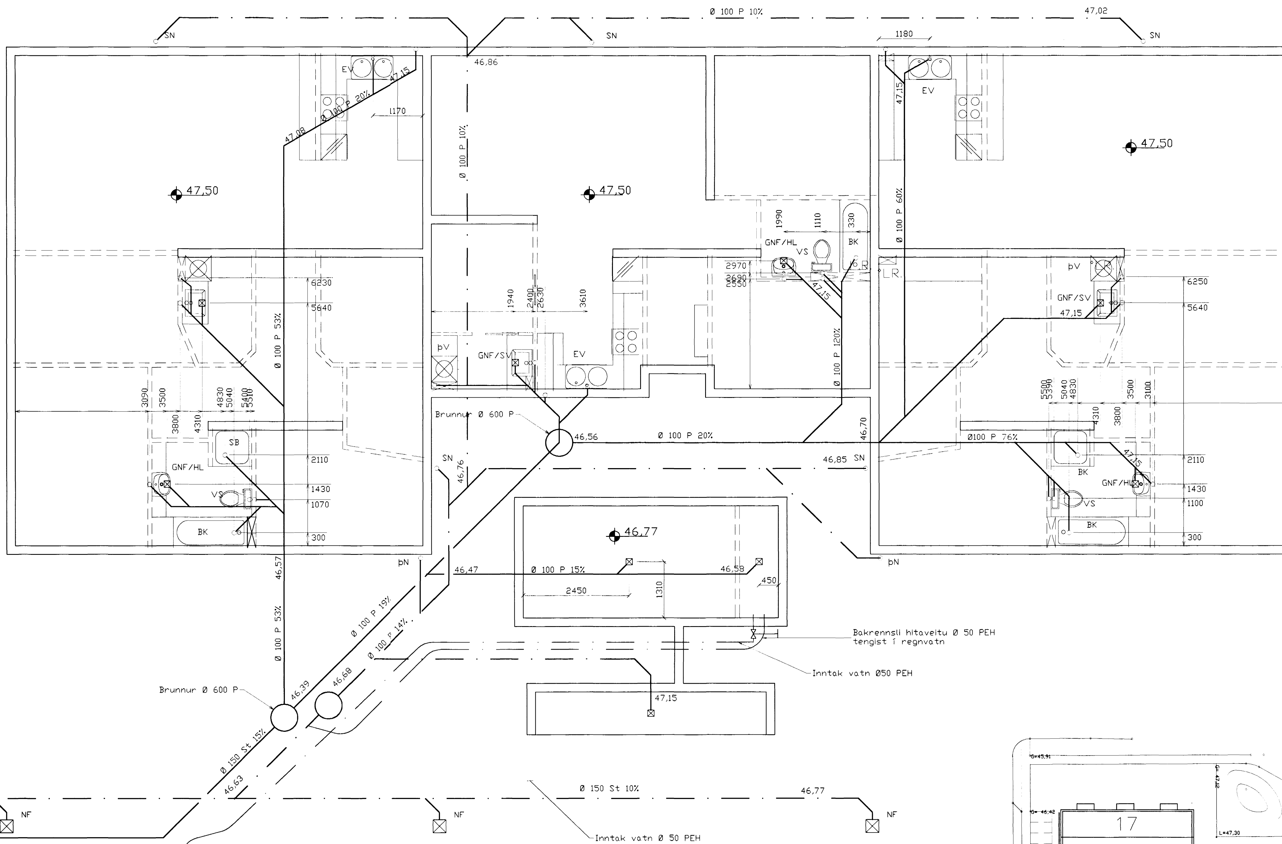
Grunnmynd 1:50
