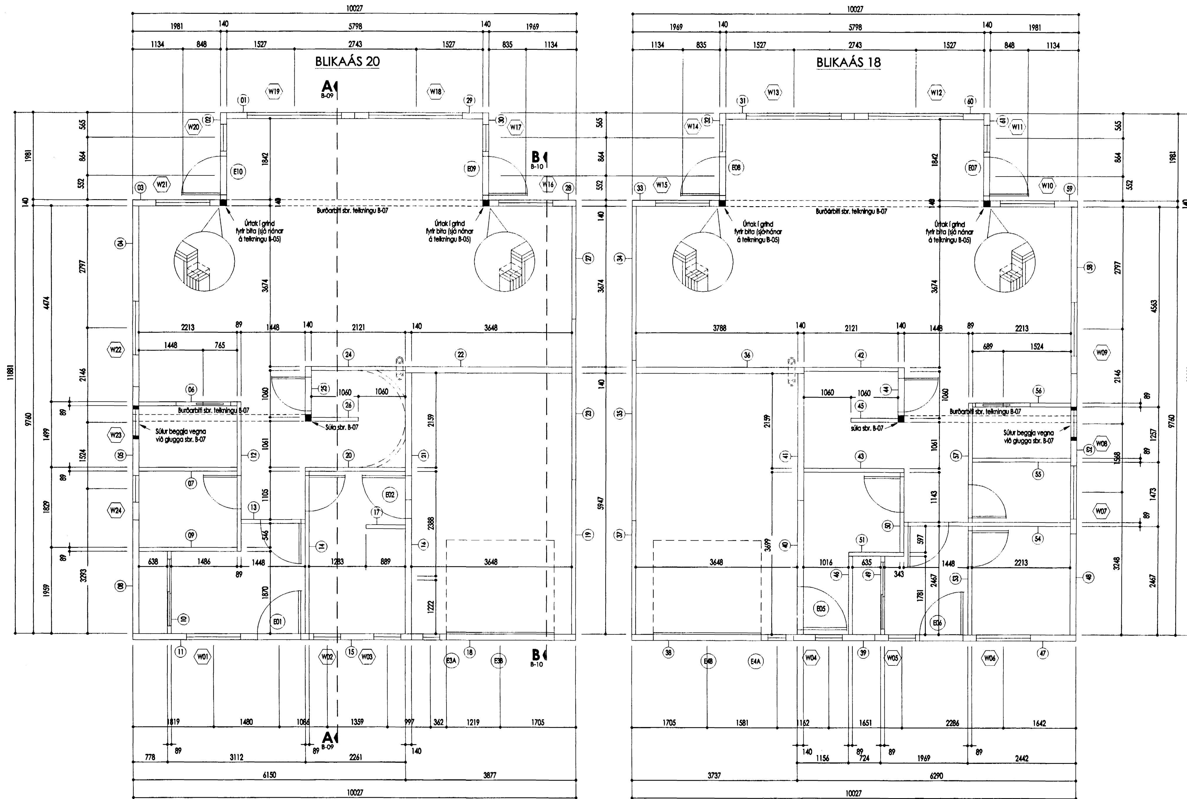
GRUNNMYND 1:50
