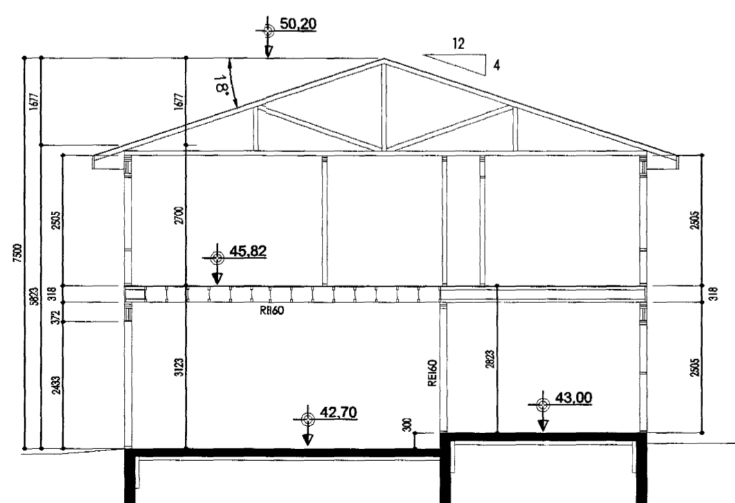
1:100 SNHD B-B
