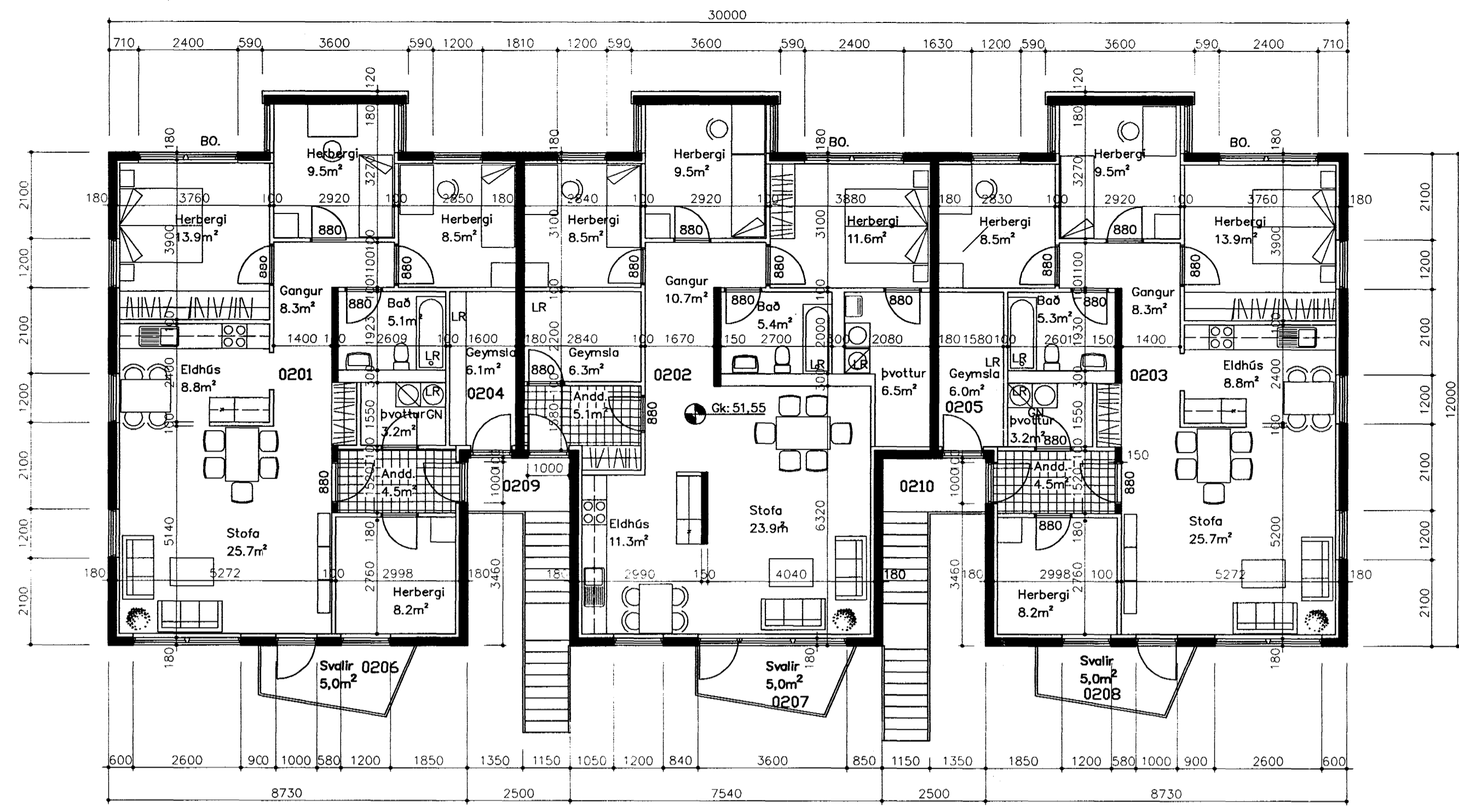
Grunnmynd 2.hæð
