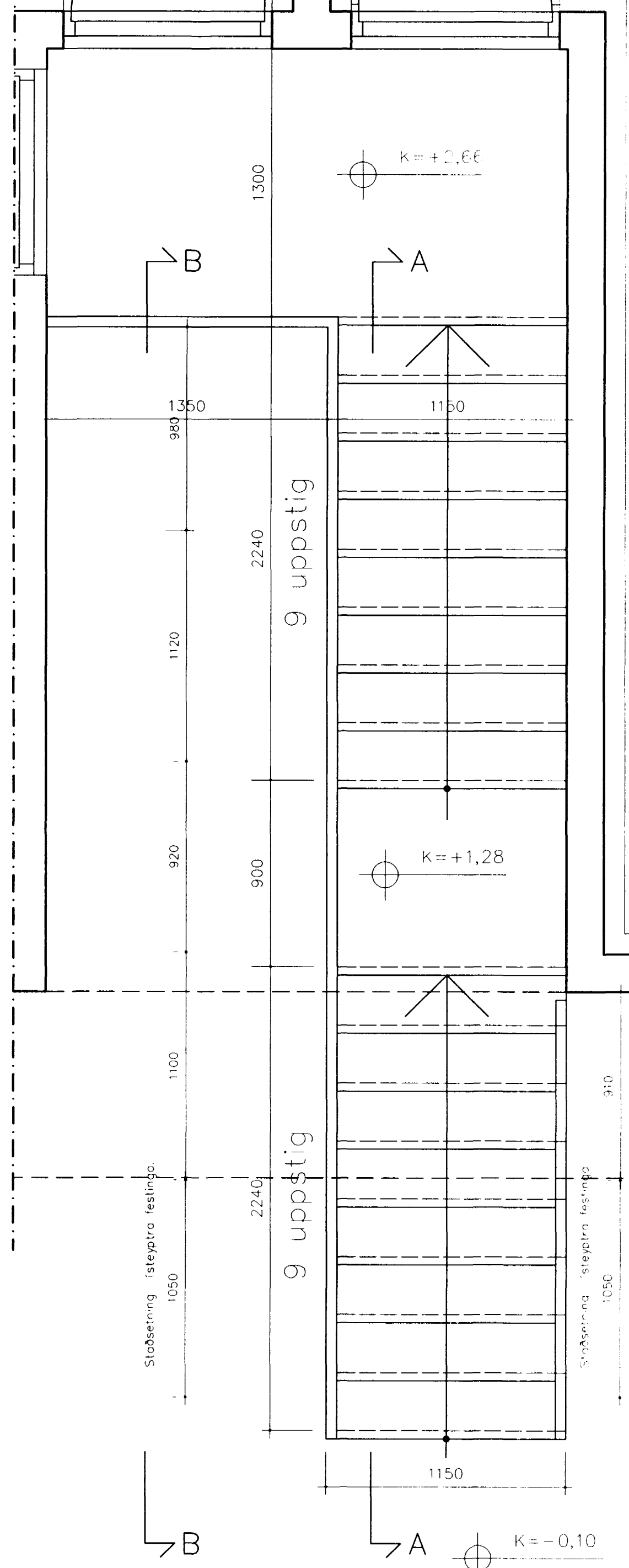
GRUNNMYND ÚTISTIGA 1:20
