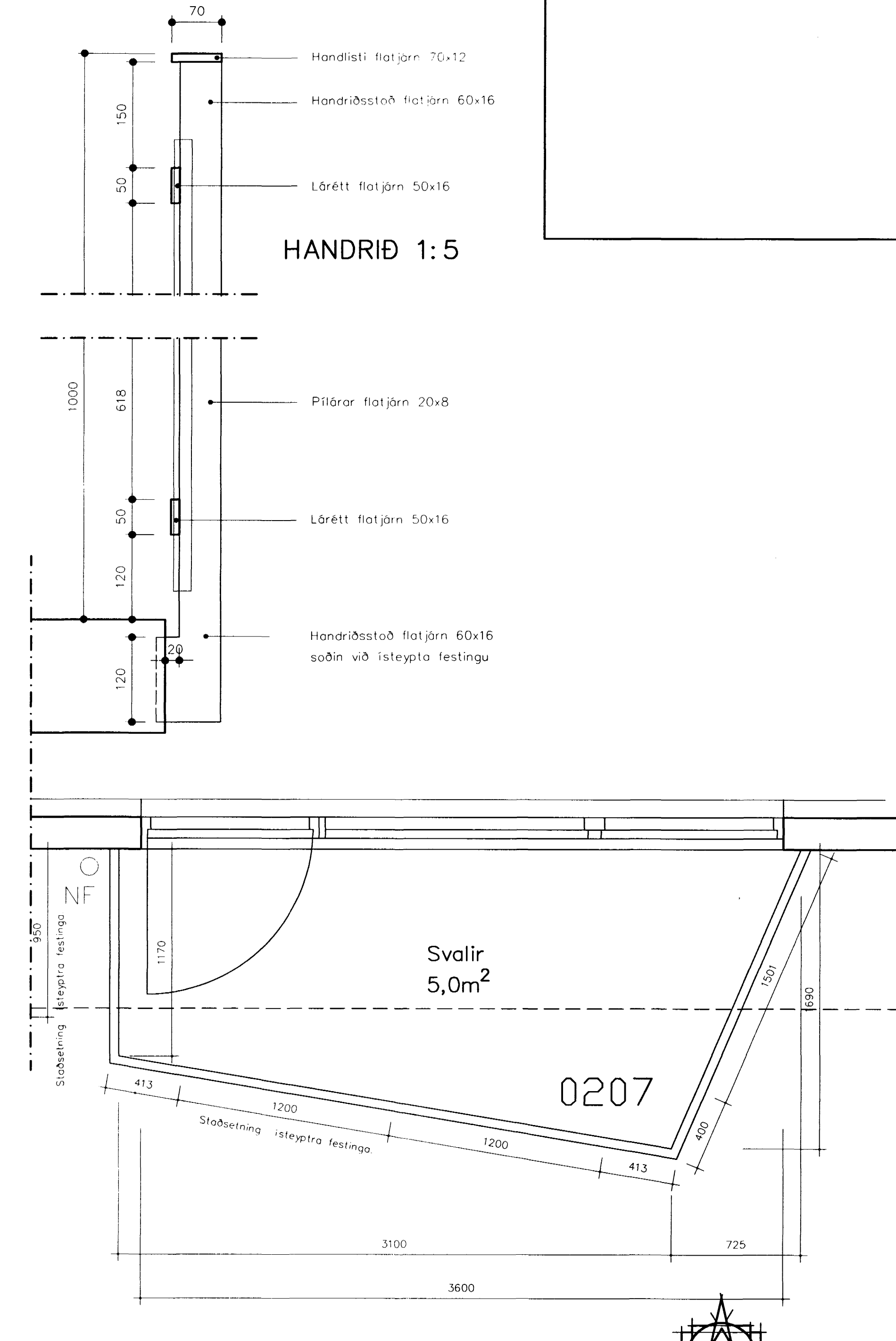
GRUNNMYND SVALA 1:20
