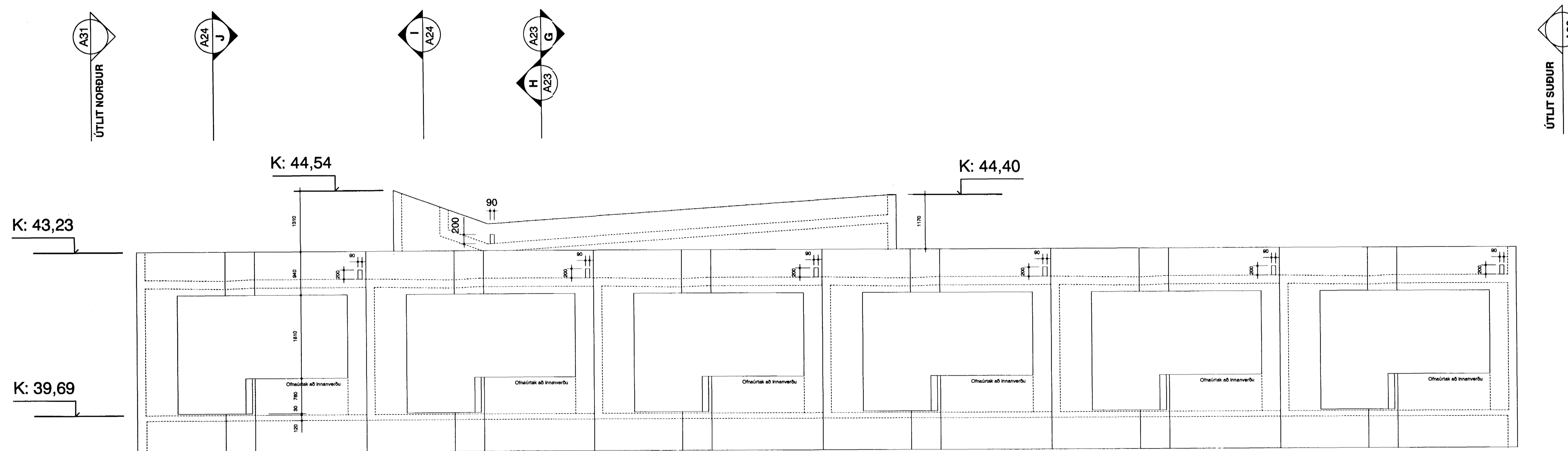
ÚTLIT VESTUR
