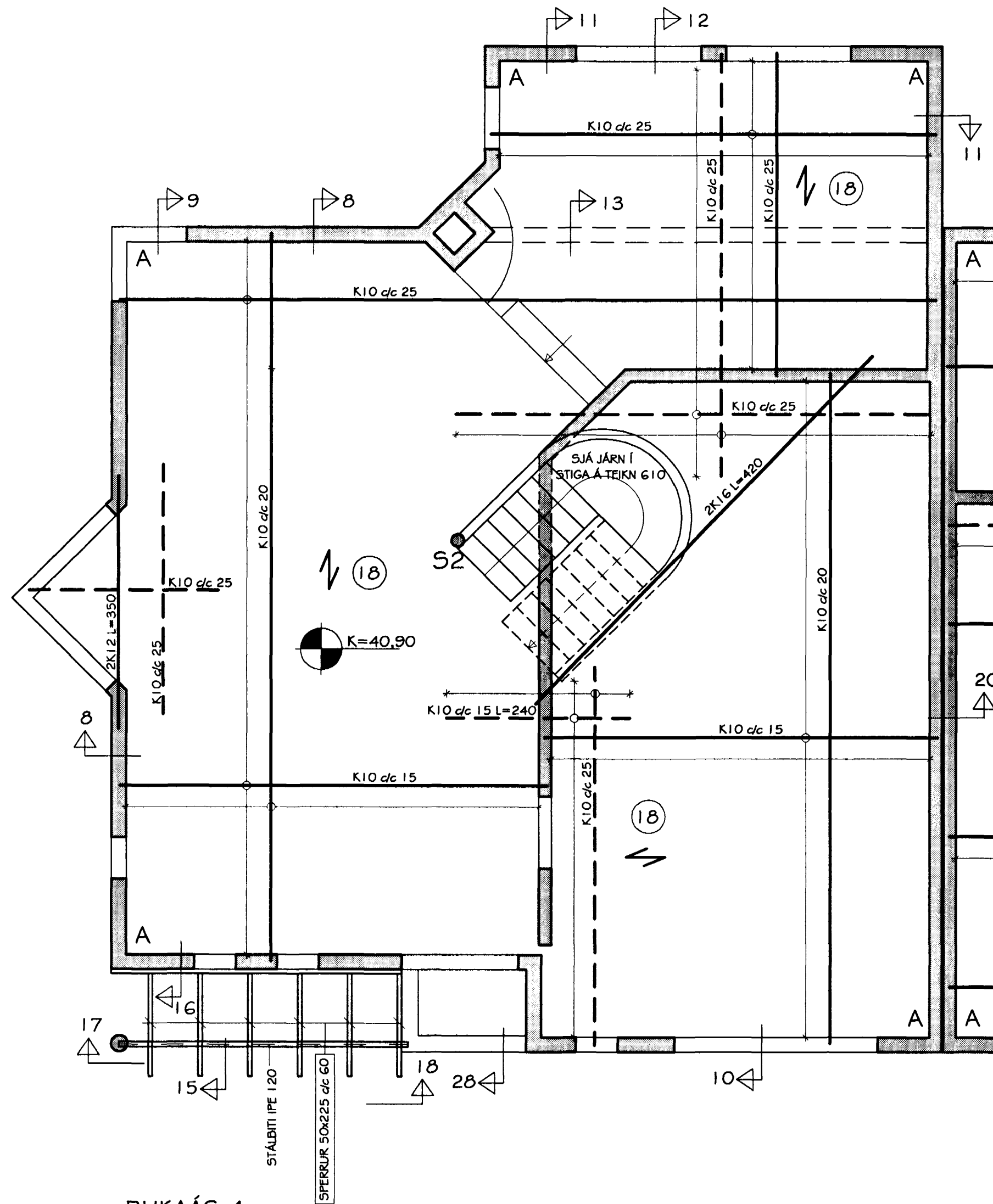
BLIKAÁS 4 JÁRN Í PLÖTU YFIR NEDRI HÆÐ GRUNNMYND MKV. 1:50
