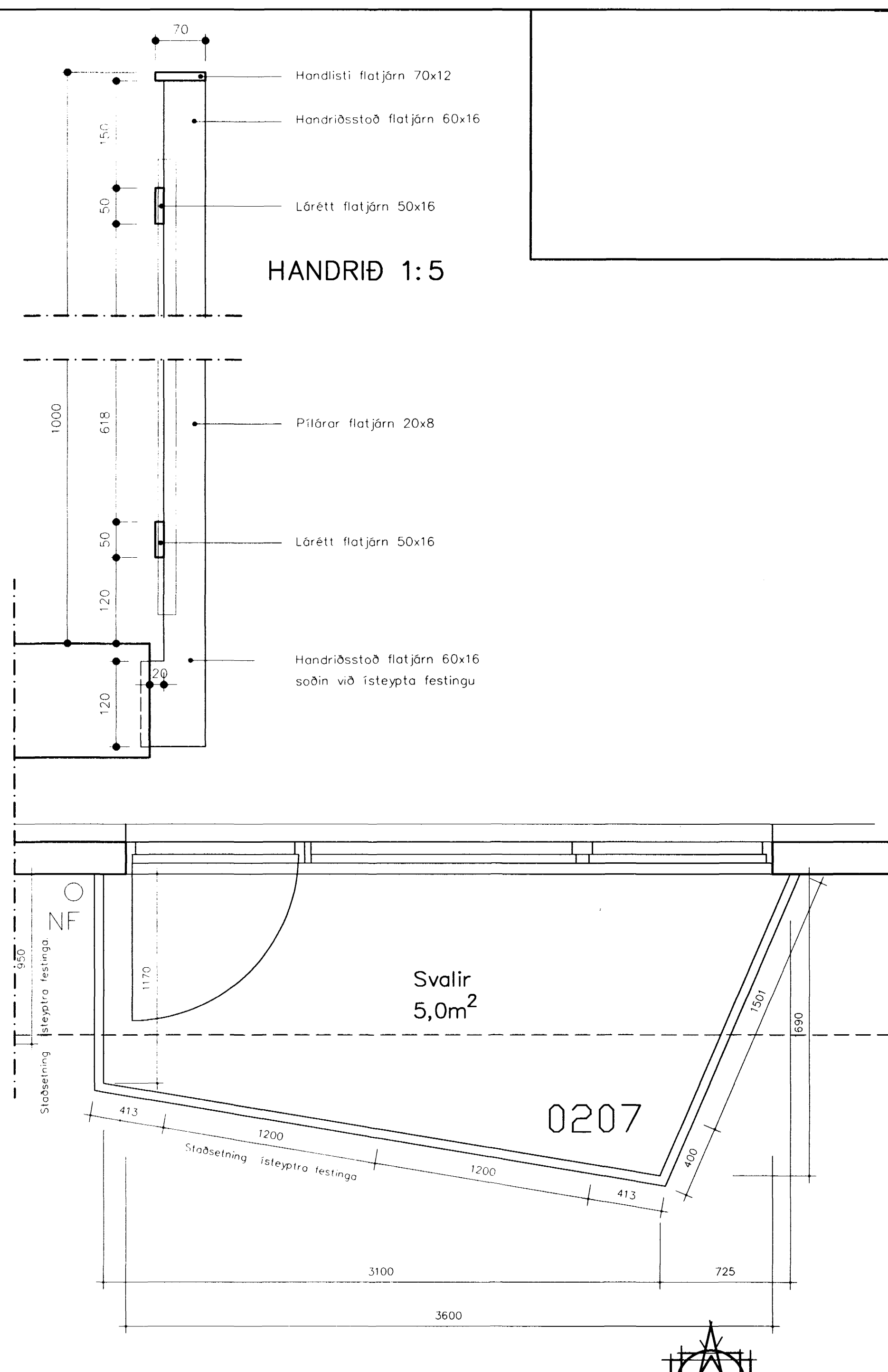
GRUNNMYND SVALA 1:20
