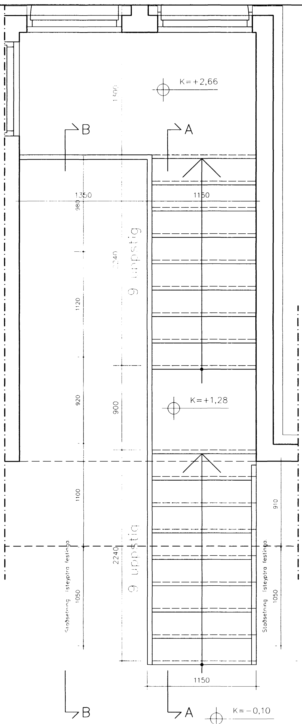
GRUNNMYND ÚTISTIGA 1:20
