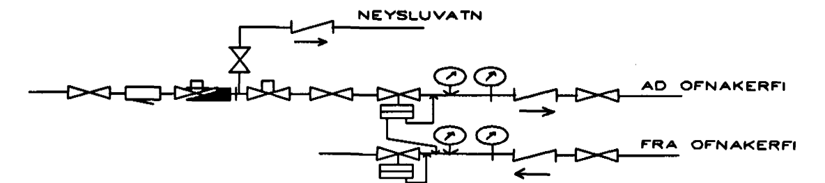
MELAGRIND HITAVEITU
