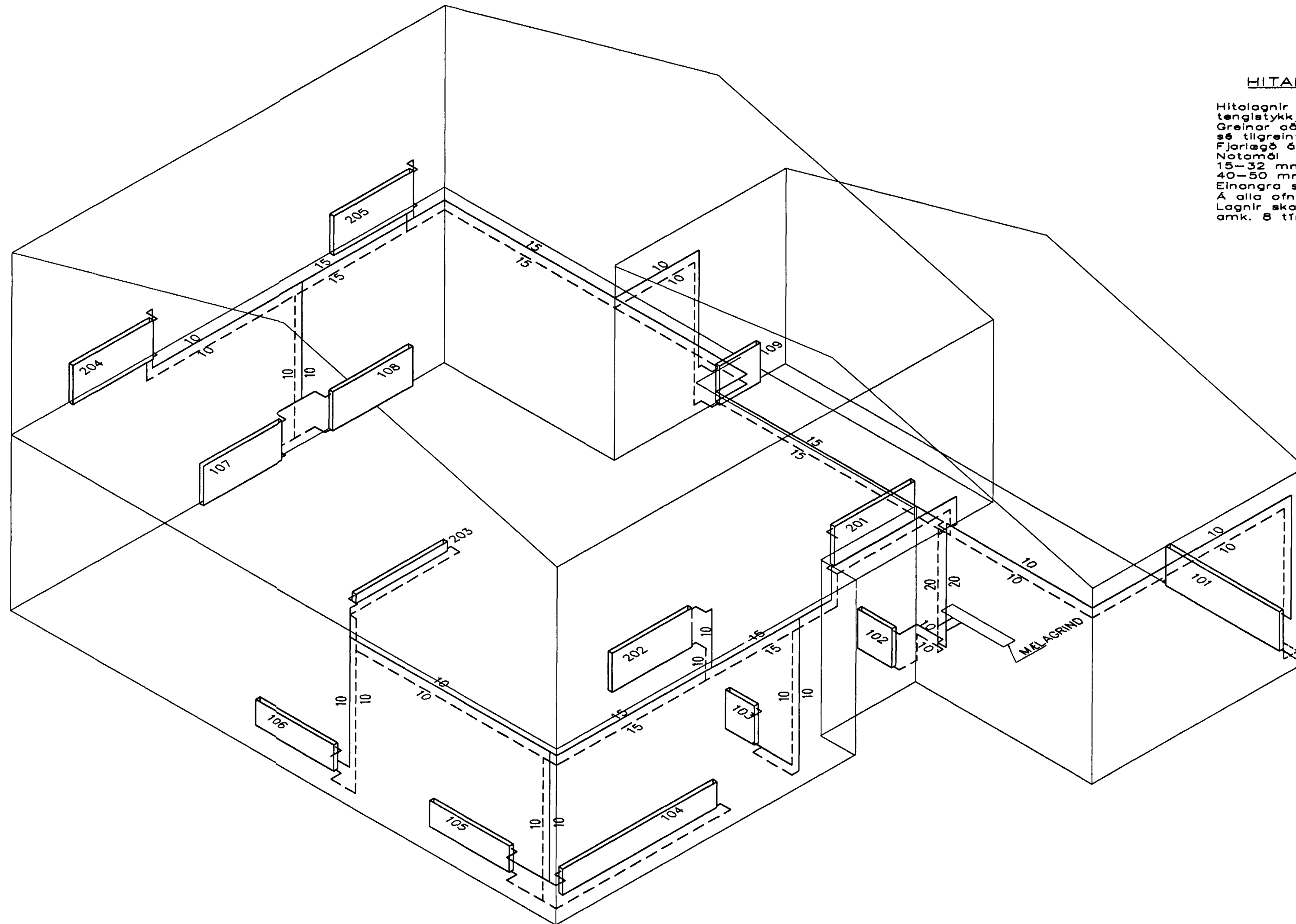
MELAGRIND HITAVEITU
