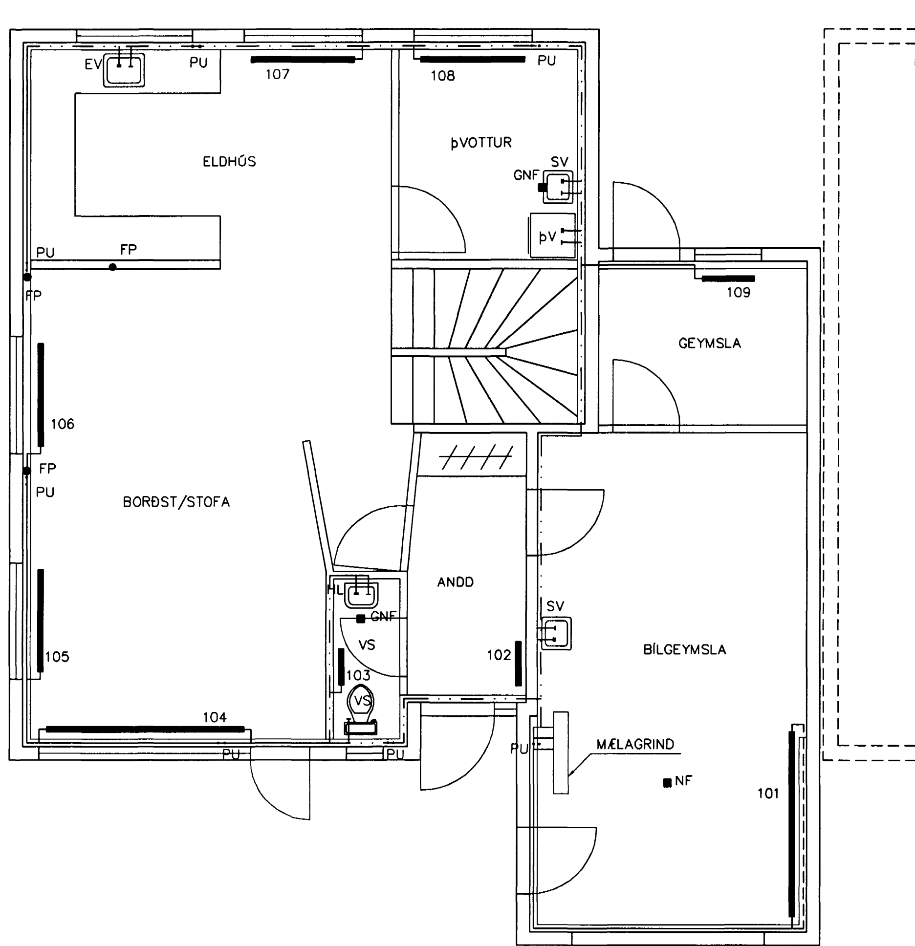
GRUNNMYND 1:50
